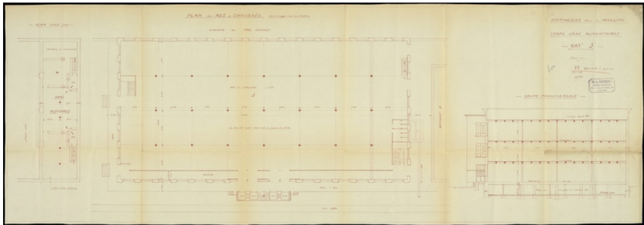
Plan bâtiment J (AC Lyon : ACL : 344 WP 1937-414., 1937, Charbon, ingénieur)
