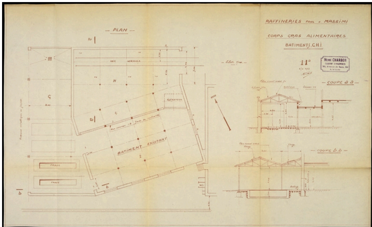
Plan bâtiment GHI (AC Lyon : Charbon ingénieur)
