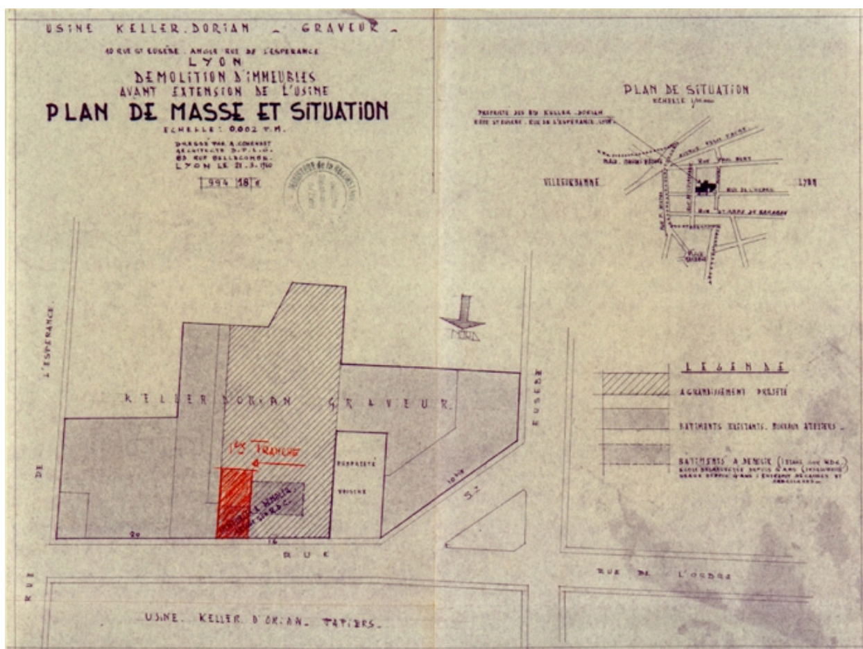
Plan de masse et situation
