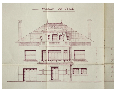
Pérignat-lès-Sarliève, la maison B.*, façade principale (détail), Jean Minot architecte, juin 1952 (Archives municipales de Pérignat-lès-Sarliève). Repro. Christophe Laurent, Autr. Jean MINOT
