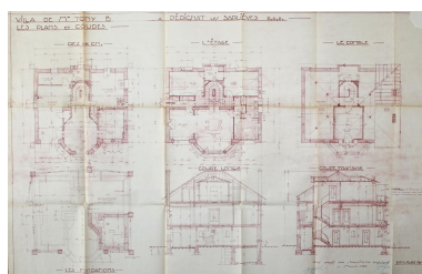
Pérignat-lès-Sarliève, la maison B.*, plans des fondations, du rez-de-chaussée, de l'étage et de l'étage de comble, Jean Minot architecte, juin 1952 (Archives municipales de Pérignat-lès-Sarliève). Repro. Christophe Laurent, Autr. Jean MINOT IVR84_2021630257NUCA
