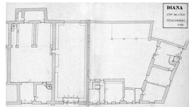
Etat des lieux, rez-de-chaussée (partie gauche) par O. Daublain et P. Hanssen, architectes, 1989. Phot. Eric Dessert, Autr. O. Daublain, Autr. P. Hanssen IVR82_20064200616NUC
