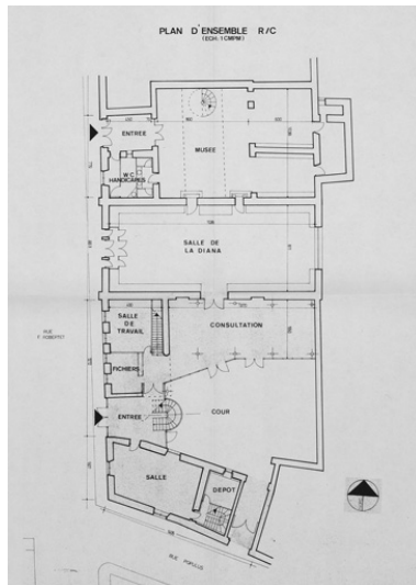
Plan d'ensemble par O. Daublain et P. Hanssen, architectes, 1989. Phot. Eric Dessert, Autr. O. Daublain, Autr. P. Hanssen IVR82_20064200628NUC
