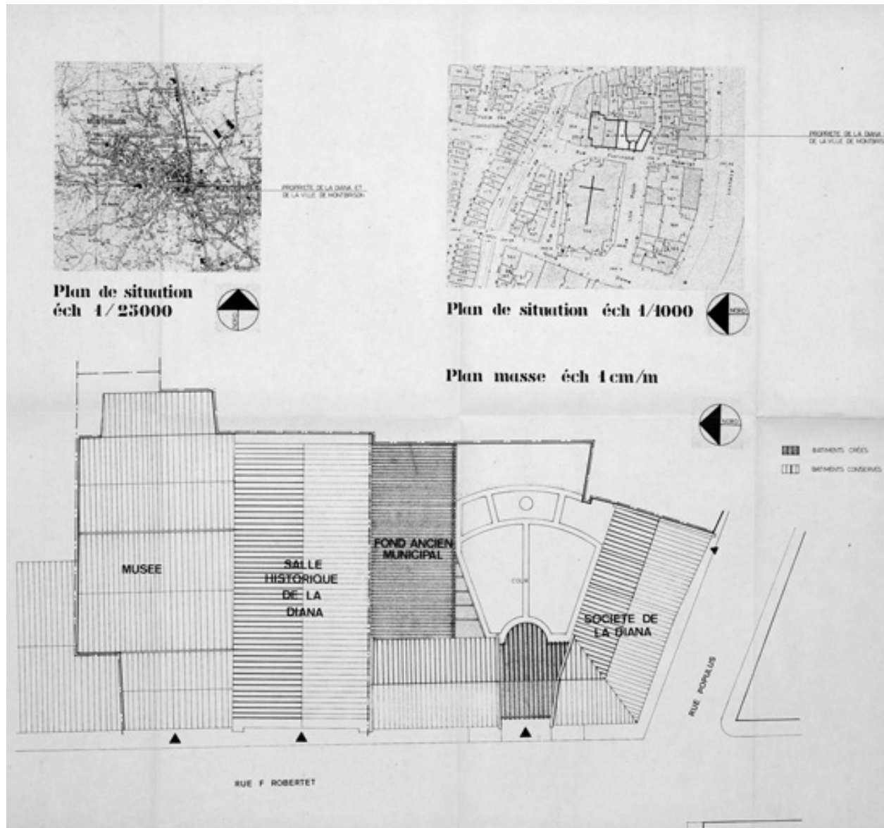
Plan de situation et plan masse. O. Daublain et P. Hanssen, architectes, 1989.
