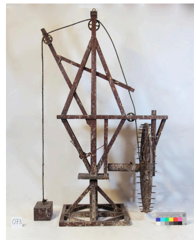
Modèle de grue, vue de face Phot. Krystelle Besson , Phot. Mirco Meier, Phot. Marion Petit IVR84_20256901115NUCA
