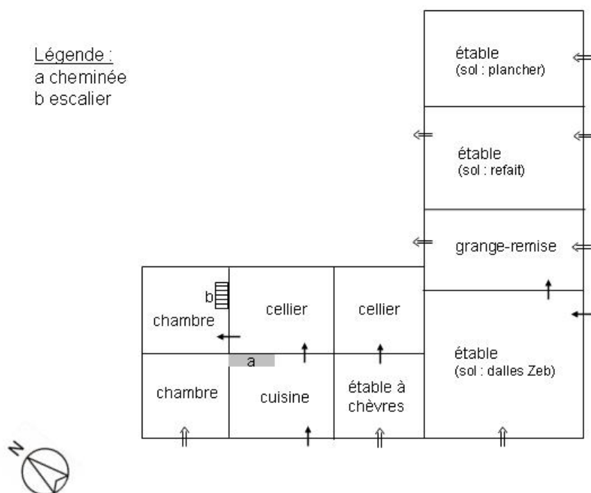
Plan schématique de la distribution du rez-de-chaussée des communs.
