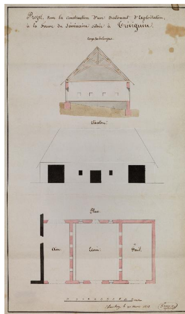
Projet pour la construction d'un bâtiment d'exploitation à la ferme du Séminaire située à Trévignin. Plan. Elévation. Coupe sur la largeur. Fournier, architecte. 1838. Phot. Thierry Leroy IVR84_20177301716NUCA
