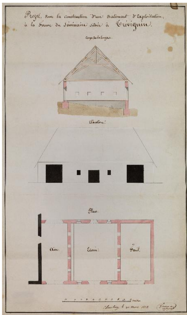
Projet pour la construction d'un bâtiment d'exploitation à la ferme du Séminaire située à Trévignin. Plan. Elévation. Coupe sur la largeur. Fournier, architecte. 1838.
