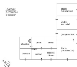
Plan schématique de la distribution du rez-de-chaussée des communs. Dess. Caroline Guibaud IVR84_20167304635NUD
