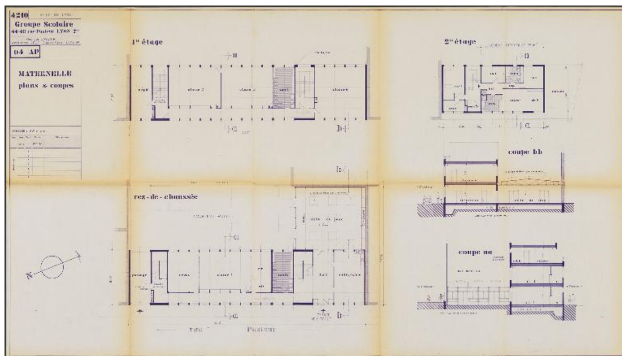
Groupe scolaire, maternelle : plans et coupes / Georges Lavenir architecte DPLG, 1970. (AC Lyon, 852 WP 004)
