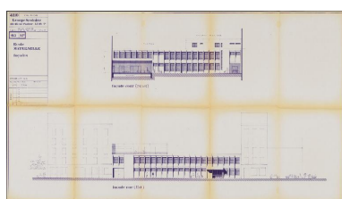
Groupe scolaire, maternelle : façades / Georges Lavenir architecte DPLG, 1970. (AC Lyon, 852 WP 004) Repro. Gilles Bernasconi, Autr. Georges Lavenir IVR84_20166901918NUCA
