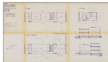
Groupe scolaire, maternelle : plans et coupes / Georges Lavenir architecte DPLG, 1970. (AC Lyon, 852 WP 004) Repro. Gilles Bernasconi, Autr. Georges Lavenir IVR84_20166901917NUCA
