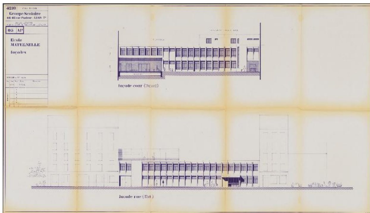
Groupe scolaire, maternelle : façades / Georges Lavenir architecte DPLG, 1970. (AC Lyon, 852 WP 004)
