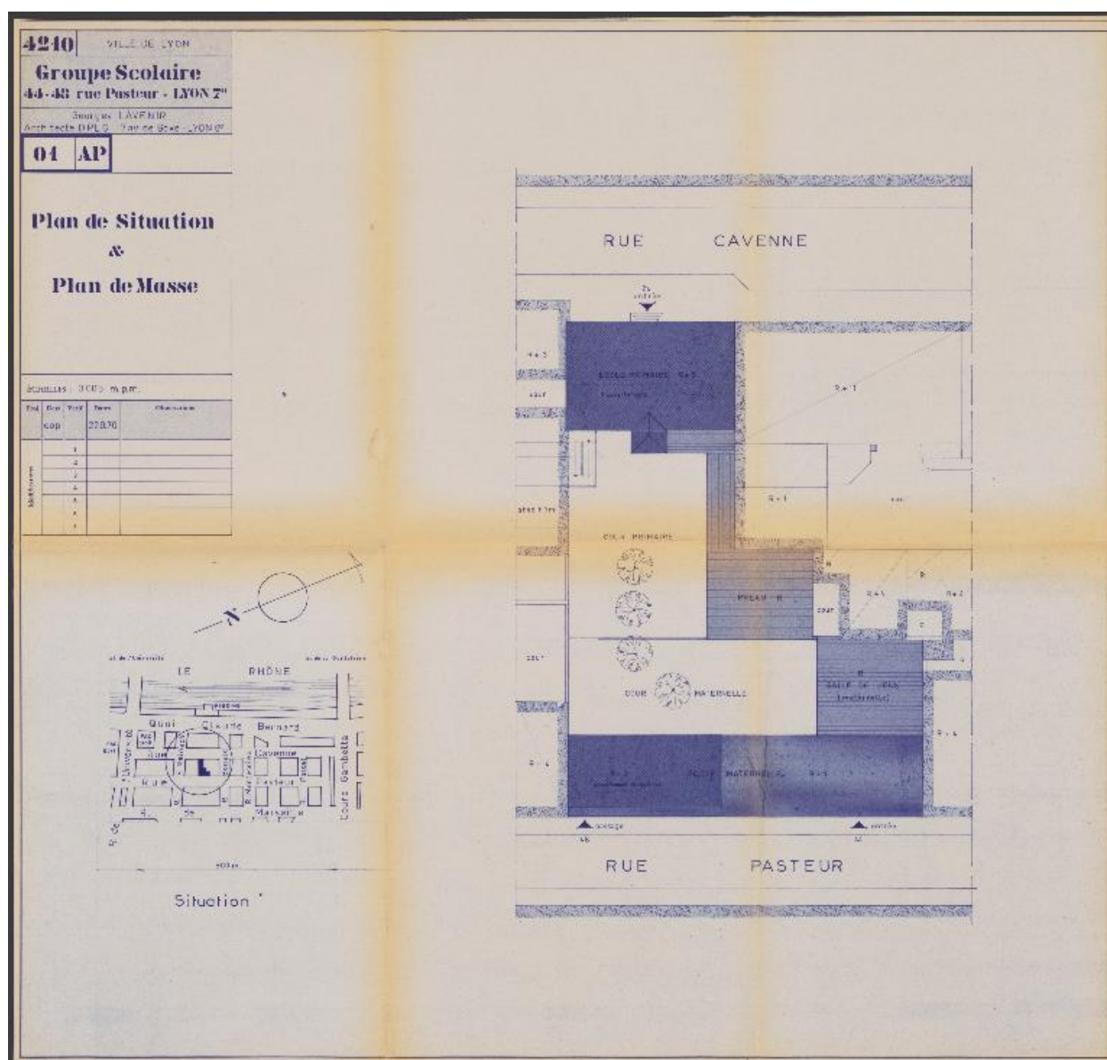
Groupe scolaire Cavenne-Pasteur. Plan de situation et plan-masse / Georges Lavenir architecte, 1972. (AC Lyon 852 WP 004)
