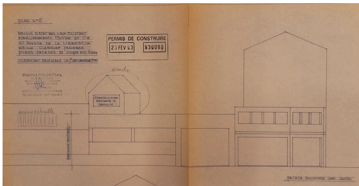
Façade sur le boulevard Jean-Jaurès
