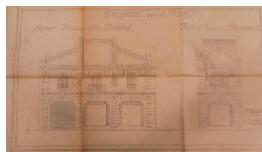
Façade et élévation latérale (projet 1927, non abouti) Repro. Félicie Fougère , Autr. Georges Laboise IVR84_20246302141NUCA
