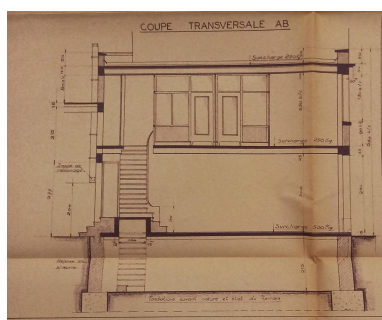
Coupe transversale Repro. Félicie Fougère , Autr. auteur inconnu IVR84_20256301324NUCA
