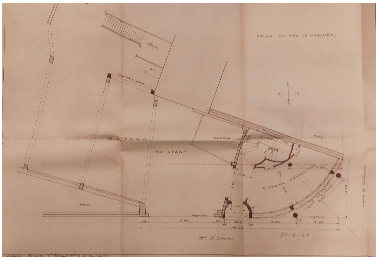
Plan du rez-de-chaussée (agrandissement 1945, projet non réalisé)
