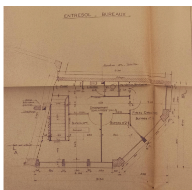
Plan de l'entresol (bureaux) Repro. Félicie Fougère , Autr. auteur inconnu IVR84_20256301323NUCA
