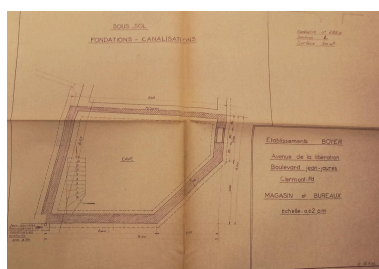
Plan du sous-sol Repro. Félicie Fougère , Autr. auteur inconnu IVR84_20256301321NUCA
