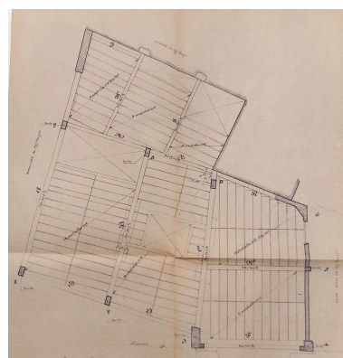
Plan des toitures, implantation du bâtiment (agrandissement 1941) Repro. Félicie Fougère IVR84_20246302147NUCA
