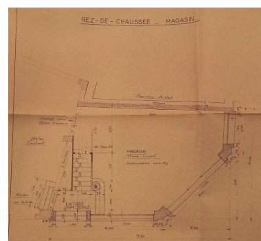
Plan du rez-de-chaussée (magasin) Repro. Félicie Fougère IVR84_20256301322NUCA
