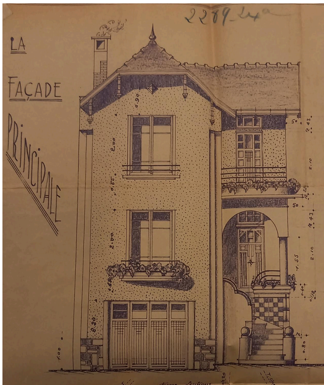
Façade, maison boulevard Josph-Girod
