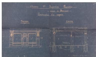
Façade sur l'avenue de Beaumont (actuelle avenue de la Libération), comparaison architecturale Repro. Félicie Fougère IVR84_20246302145NUCA
