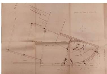
Plan du rez-de-chaussée (agrandissement 1945, projet non réalisé) Repro. Félicie Fougère , Autr. Valentin Vigneron IVR84_20246302152NUCA
