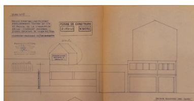
Façade sur le boulevard Jean-Jaurès Repro. Félicie Fougère , Autr. Pierre Courtial IVR84_20256301328NUCA
