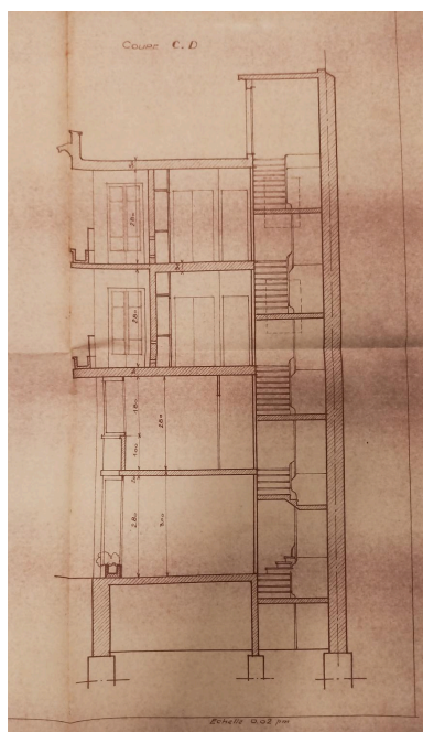
Coupe longitudinale (agrandissement 1945, projet non réalisé) Repro. Félicie Fougère , Autr. Valentin Vigneron IVR84_20246302151NUCA
