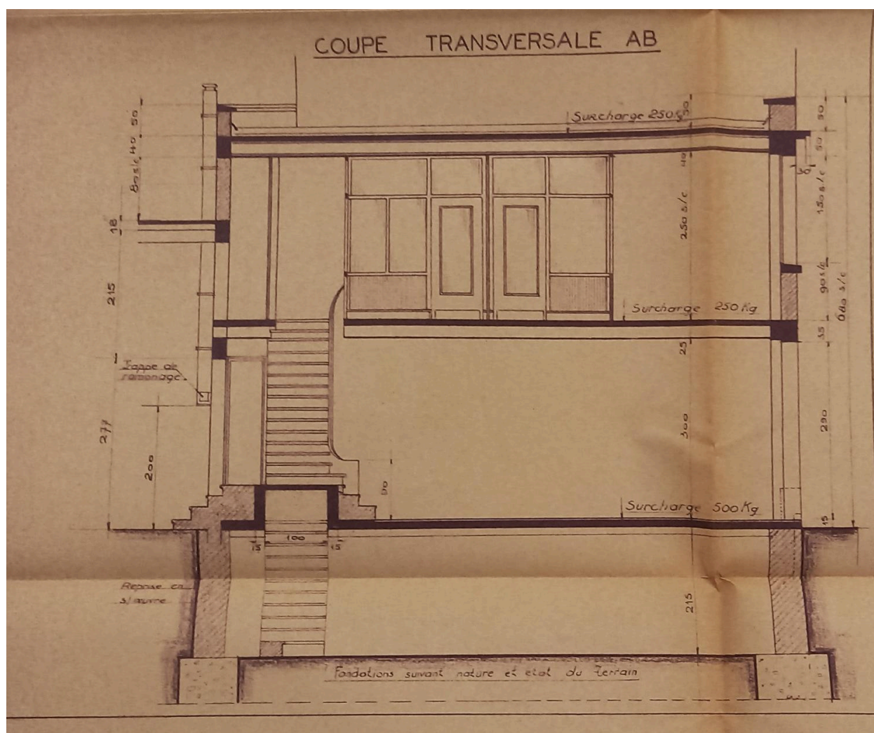
Coupe transversale
