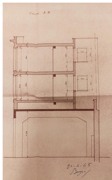
Coupe transversale (agrandissement 1945, projet non réalisé) Repro. Félicie Fougère , Autr. Valentin Vigneron IVR84_20246302150NUCA
