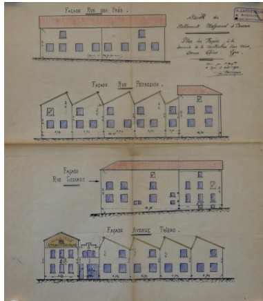
Façades des Ets Maljournal et Bourron, 1910, Lyon 6e ((AC Lyon 314W/397-548) Phot. Nadine Halitim-Dubois IVR84_20246900700NUCA
