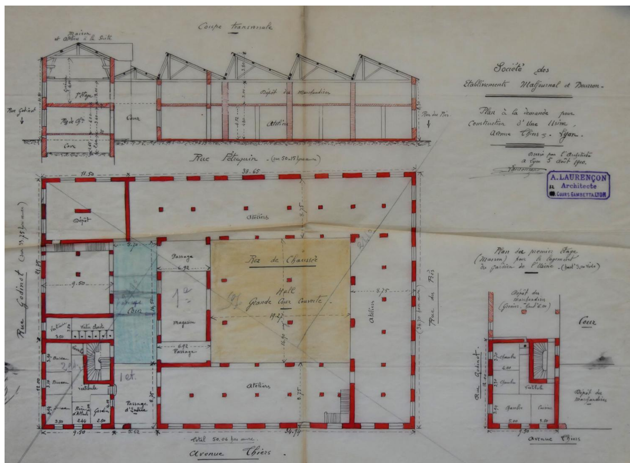
Coupe transversale et plan du rez-de-chaussée Ets Maljournal et Bourron 1910 (AC Lyon 314W/480)
