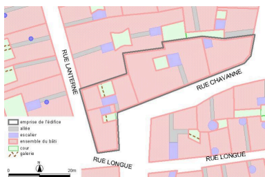
Plan-masse, d'après le système urbain de référence, version 1999 Dess. Paul Cherblanc IVR82_20056902702NUDA
