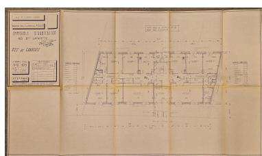
Plan du rez-de-chaussée surélevé de l'immeuble. Repro. Brigitte Ceroni, Autr. auteur inconnu IVR84_20256301439NUCA
