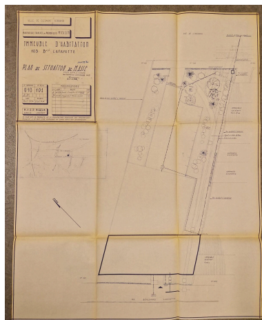
Plan de situation et plan masse de l'immeuble. Repro. Brigitte Ceroni, Autr. auteur inconnu IVR84_20256301437NUCA
