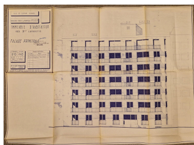
Élévation principale de l'immeuble sur le boulevard Lafayette. Repro. Brigitte Ceroni, Autr. auteur inconnu IVR84_20256301443NUCA
