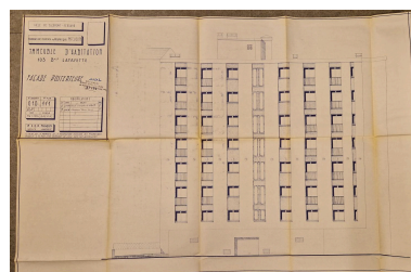
Élévation postérieure de l'immeuble. Repro. Brigitte Ceroni, Autr. auteur inconnu IVR84_20256301444NUCA
