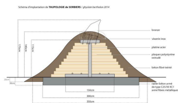
Schéma d'implantation. Phot. Ghyslain Bertholon IVR84_20204200124NUCAB
