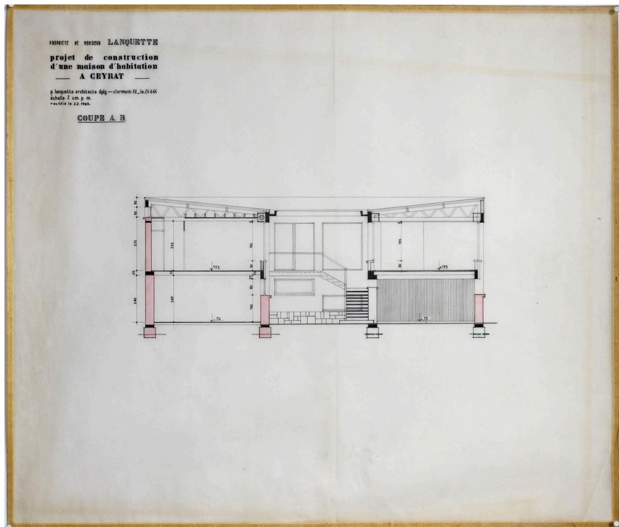
Ceyrat, la maison L., coupe A-B, 24 juin 1964, Paul Lanquette architecte (archives privées famille Lanquette).
