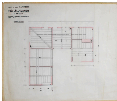
Ceyrat, la maison L., plan de la charpente, 24 juin 1964, Paul Lanquette architecte (archives privées famille Lanquette). Repro. Christophe Laurent, Autr. Paul Lanquette IVR84_20216302573NUCA
