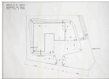
Ceyrat, la maison L., plan d'aménagement des abords, 15 octobre 1965, Paul Lanquette architecte (archives privées famille Lanquette). Repro. Christophe Laurent, Autr. Paul Lanquette IVR84_20216302570NUCA
