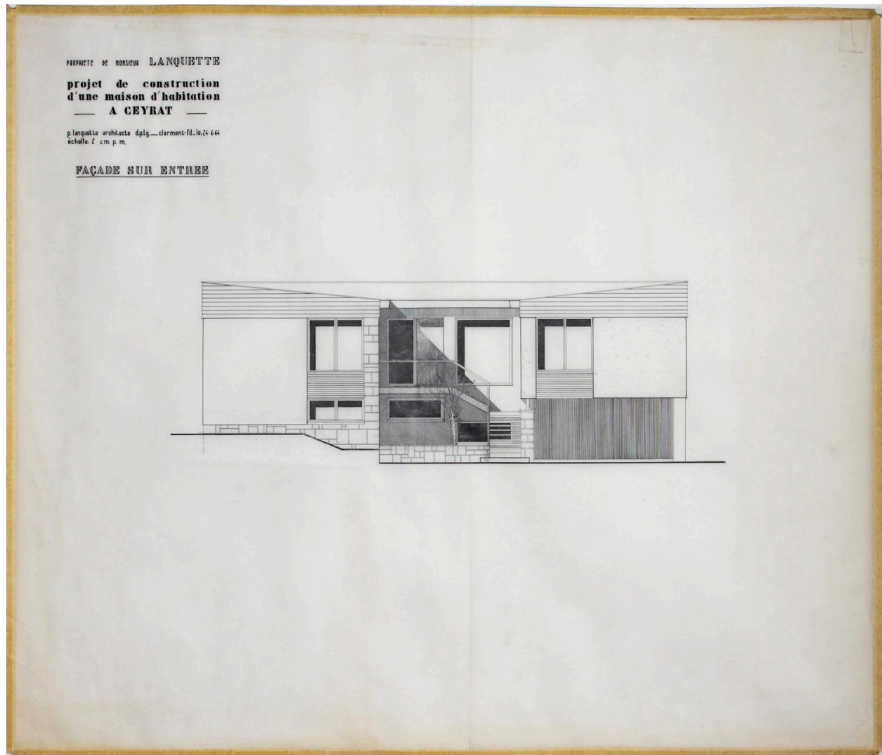
Ceyrat, la maison L., façade principale (sud), 24 juin 1964, Paul Lanquette architecte (archives privées famille Lanquette).
