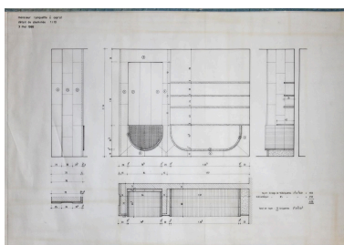
Ceyrat, la maison L., plan et élévation du foyer, du manteau et du coffre de la cheminée du séjour, 3 mai 1966, Paul Lanquette architecte (archives privées famille Lanquette). Repro. Christophe Laurent, Autr. Paul Lanquette IVR84_20216302579NUCA
