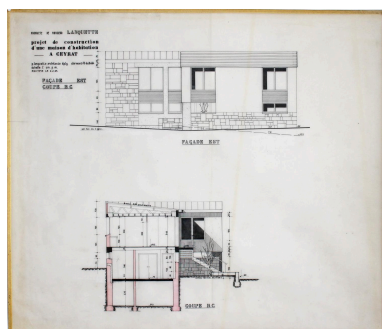
Ceyrat, la maison L., façades est et coupe B-C, 24 juin 1964, Paul Lanquette architecte (archives privées famille Lanquette). Repro. Christophe Laurent, Autr. Paul Lanquette IVR84_20216302575NUCA
