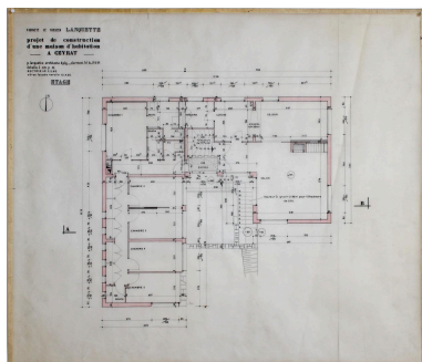
Ceyrat, la maison L., plan de l'étage, 24 juin 1964, Paul Lanquette architecte (archives privées famille Lanquette). Repro. Christophe Laurent, Autr. Paul Lanquette IVR84_20216302572NUCA
