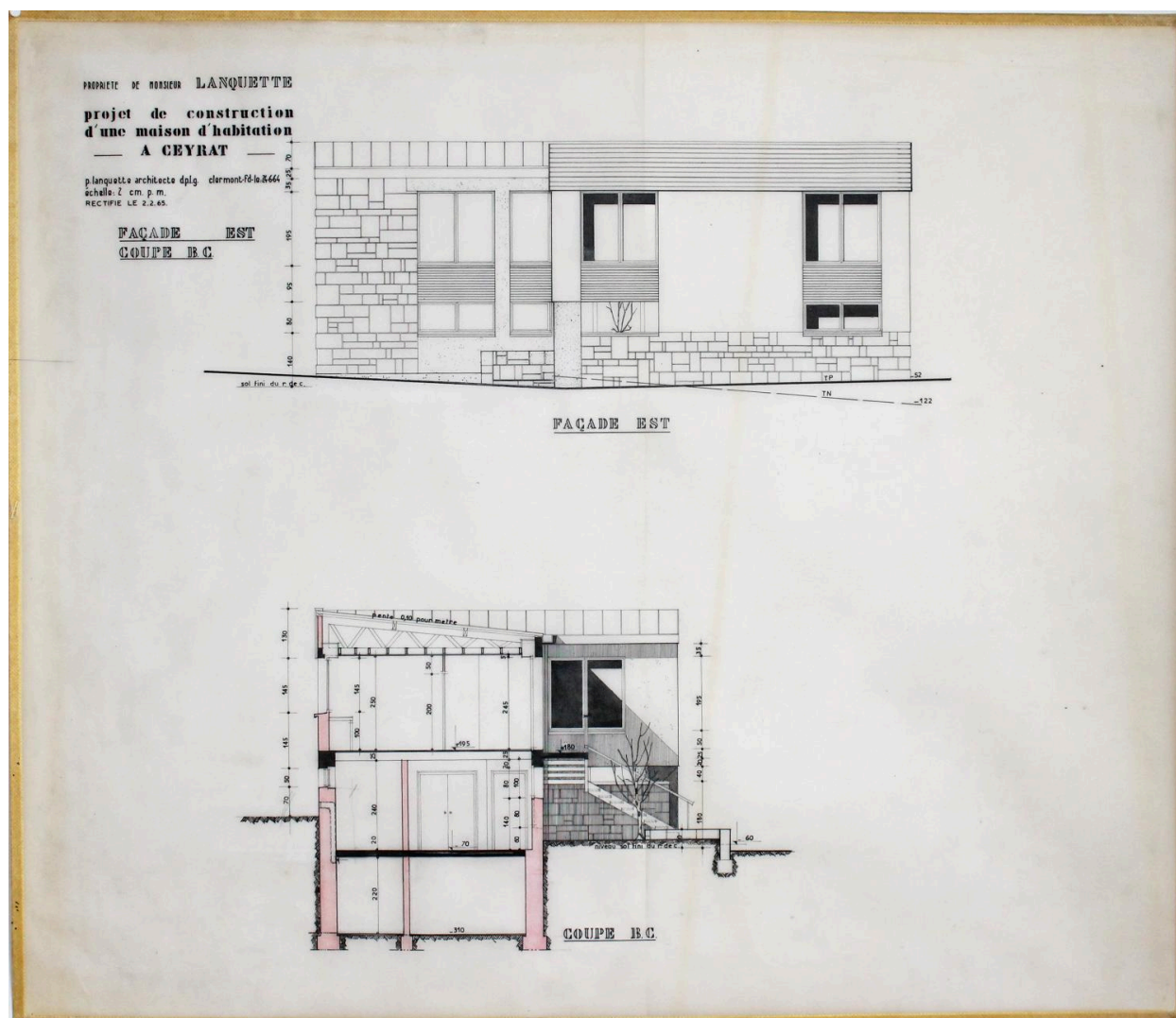
Ceyrat, la maison L., façades est et coupe B-C, 24 juin 1964, Paul Lanquette architecte (archives privées famille Lanquette).
