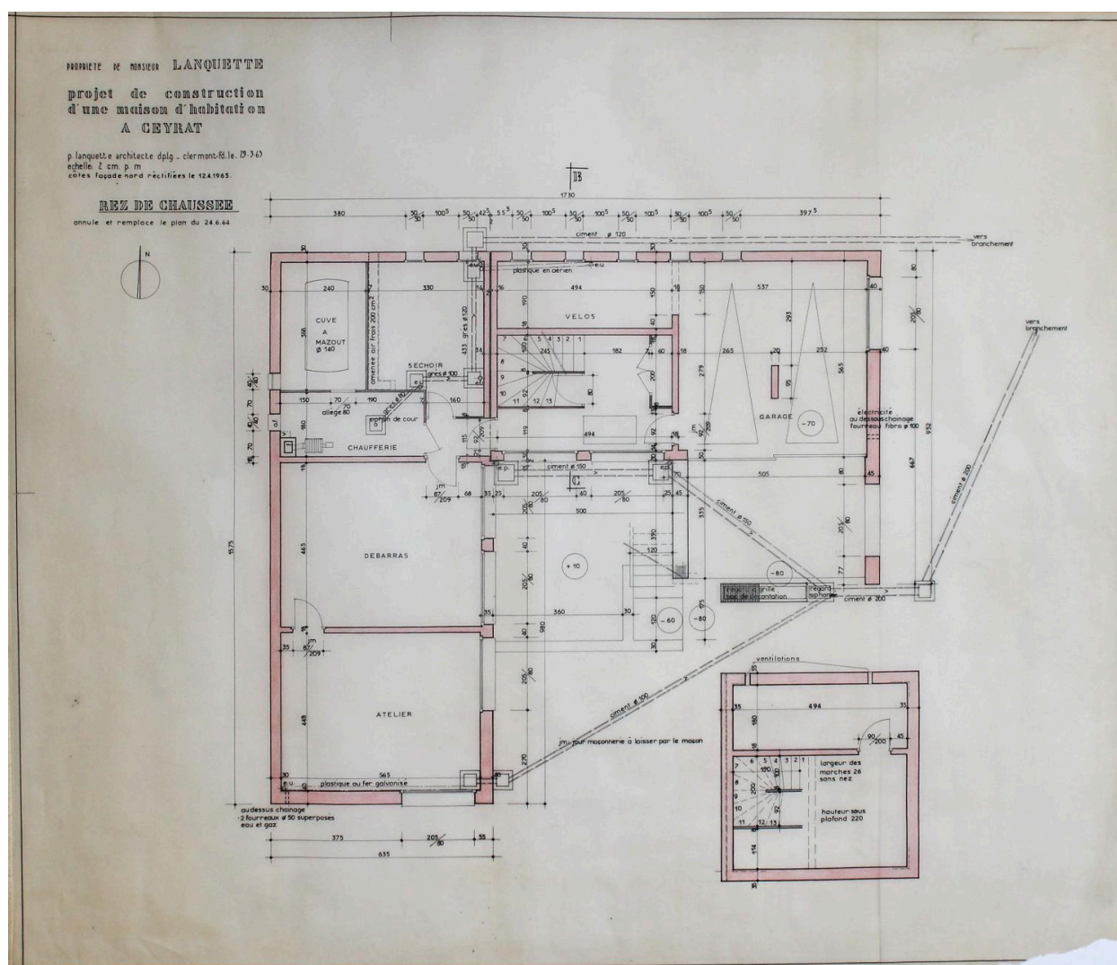
Ceyrat, la maison L., plan du rez-de-chaussée, 29 mars 1965, Paul Lanquette architecte (archives privées famille Lanquette).
