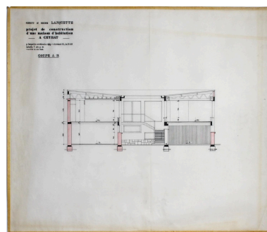
Ceyrat, la maison L., coupe A-B, 24 juin 1964, Paul Lanquette architecte (archives privées famille Lanquette). Repro. Christophe Laurent, Autr. Paul Lanquette IVR84_20216302577NUCA
