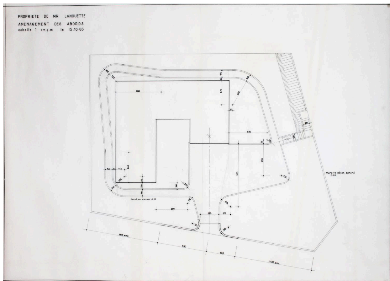
Ceyrat, la maison L., plan d'aménagement des abords, 15 octobre 1965, Paul Lanquette architecte (archives privées famille Lanquette).
