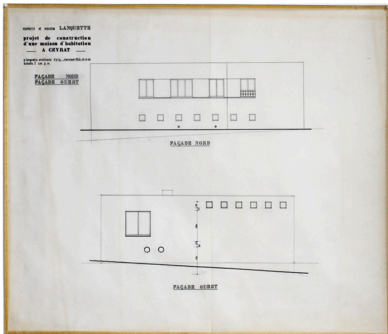
Ceyrat, la maison L., façades nord et ouest, 24 juin 1964, Paul Lanquette architecte (archives privées famille Lanquette).
