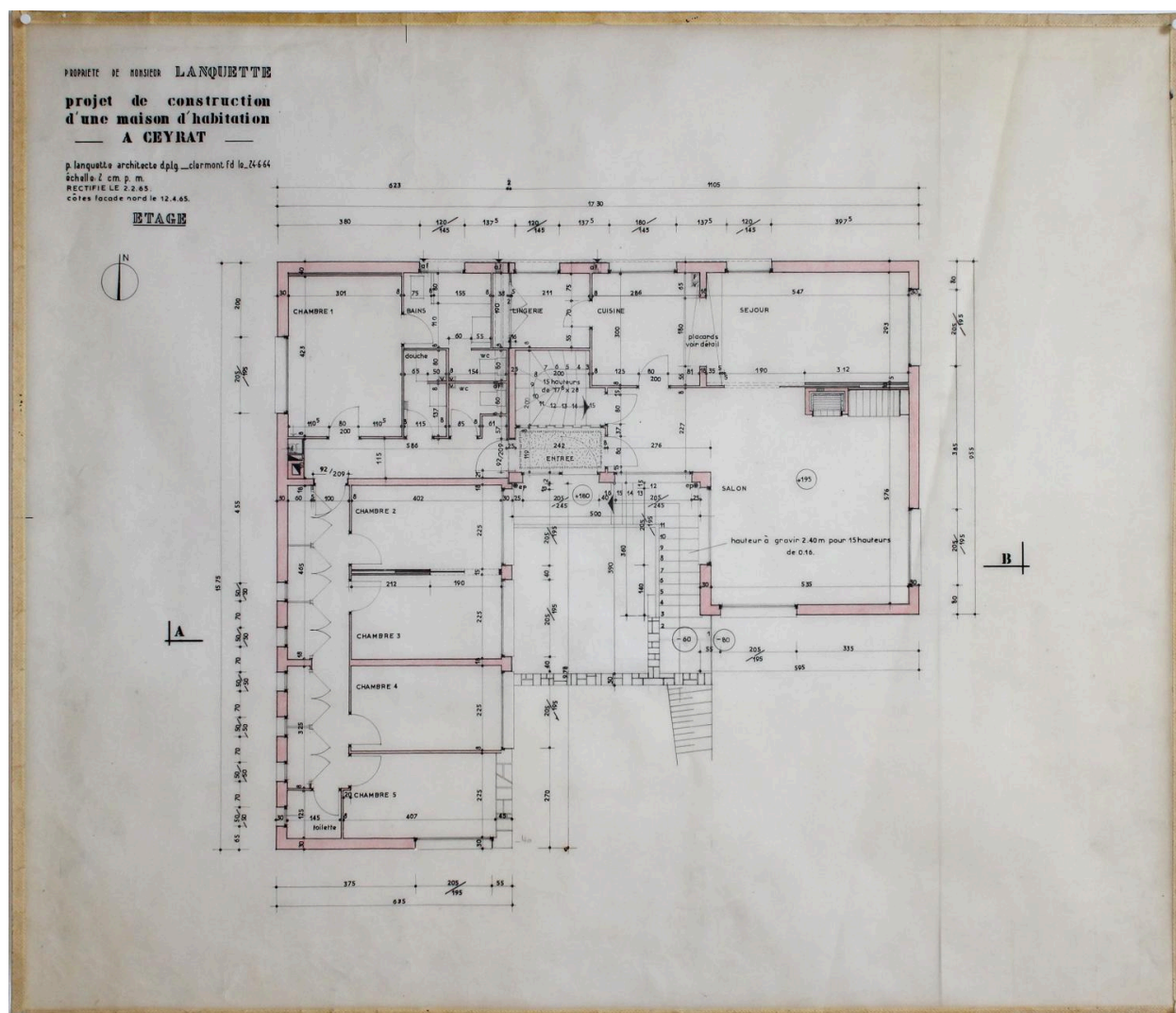
Ceyrat, la maison L., plan de l'étage, 24 juin 1964, Paul Lanquette architecte (archives privées famille Lanquette).
