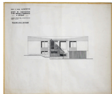
Ceyrat, la maison L., façade principale (sud), 24 juin 1964, Paul Lanquette architecte (archives privées famille Lanquette). Repro. Christophe Laurent, Autr. Paul Lanquette IVR84_20216302574NUCA
