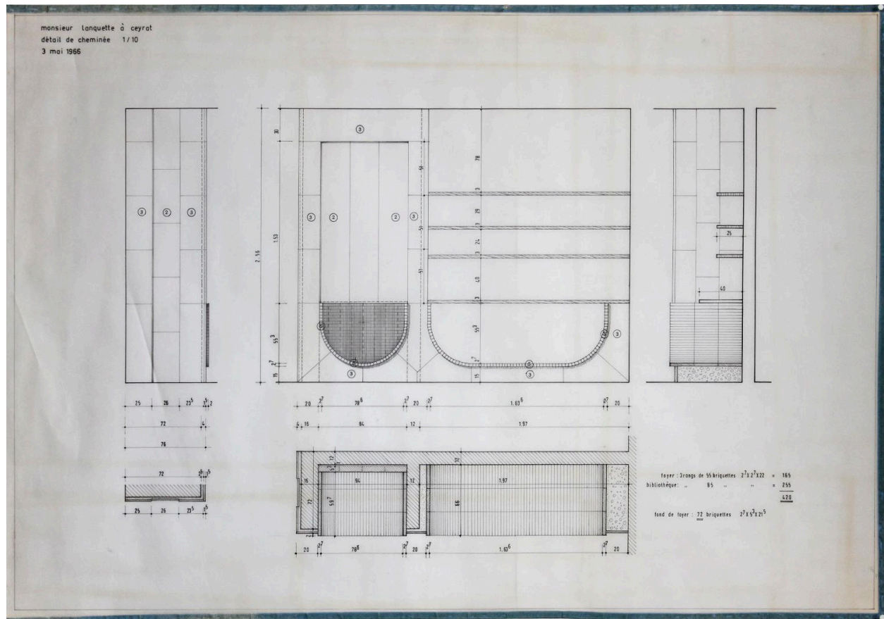
Ceyrat, la maison L., plan et élévation du foyer, du manteau et du coffre de la cheminée du séjour, 3 mai 1966, Paul Lanquette architecte (archives privées famille Lanquette).
