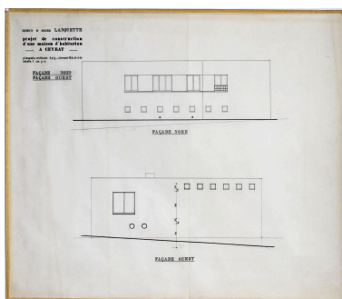
Ceyrat, la maison L., façades nord et ouest, 24 juin 1964, Paul Lanquette architecte (archives privées famille Lanquette). Repro. Christophe Laurent, Autr. Paul Lanquette IVR84_20216302576NUCA
