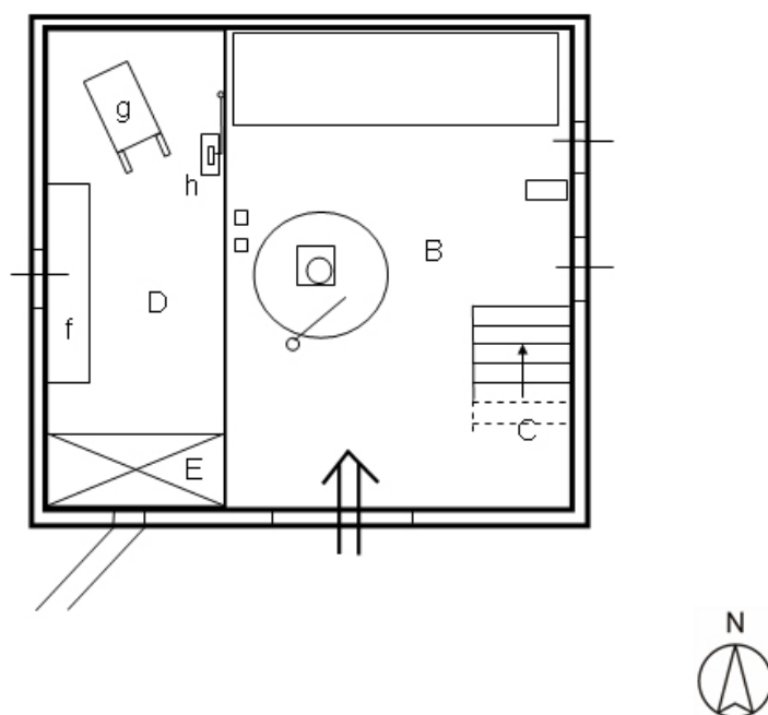
Plan de masse et de situation du rez-de-chaussée surélevé avec plateforme surélevée
