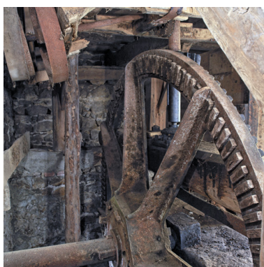
Moulin, étage de soubassement, vue d'ensemble du mécanisme. Phot. Didier Gourbin IVR82_20064200836NUCA
