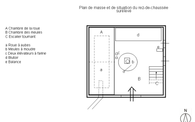
Plan de masse et de situation du rez-de-chaussée surélevé avec roue à aubes. Dess. Thierry Monnet IVR82_20124200515NUD
