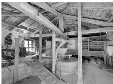
Rez-de-chaussée surélevé, vue d'ensemble de la salle de mouture. Phot. Didier Gourbin IVR82_20064200804V
