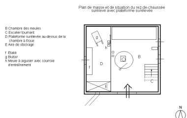
Plan de masse et de situation du rez-de-chaussée surélevé avec plateforme. Dess. Thierry Monnet IVR82_20124200516NUD
