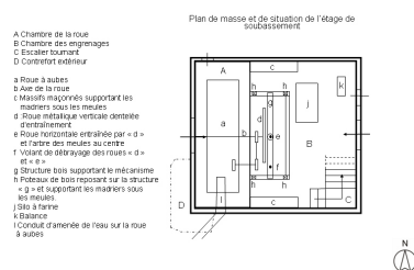
Plan de masse et de situation de l'étage de soubassement du moulin. Dess. Thierry Monnet IVR82_20124200514NUD
