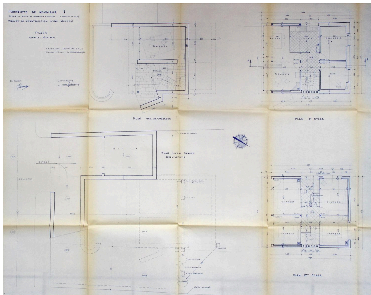
Durtol, la Maison I., plans des niveaux, 1959, Antoine Espinasse architecte (Archives municipales de Durtol).
