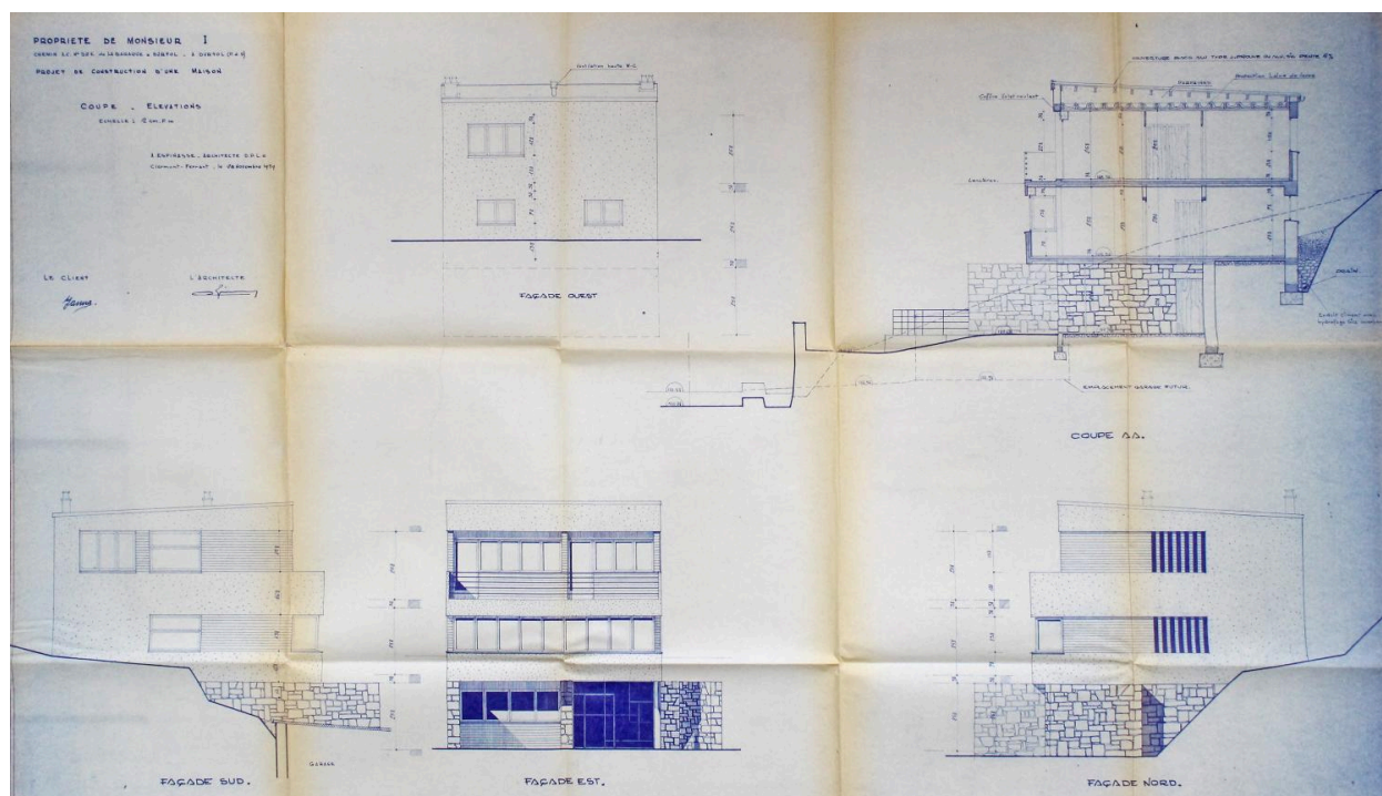
Durtol, la Maison I., coupe et élévations, 1959, Antoine Espinasse architecte (Archives municipales de Durtol).
