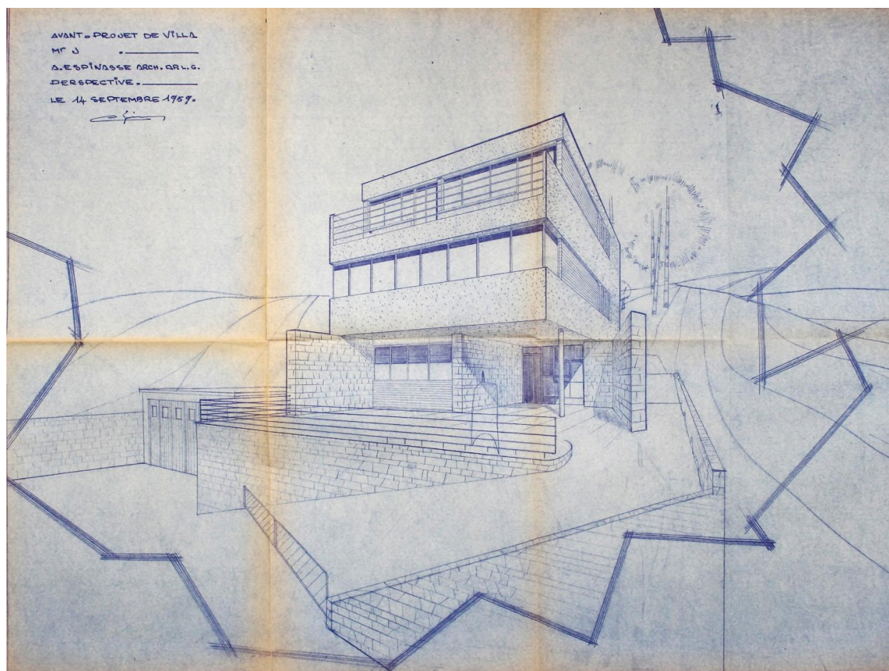
Durtol, la Maison I., élévation en perspective, avant-projet, 1959, Antoine Espinasse architecte (Archives municipales de Durtol).
