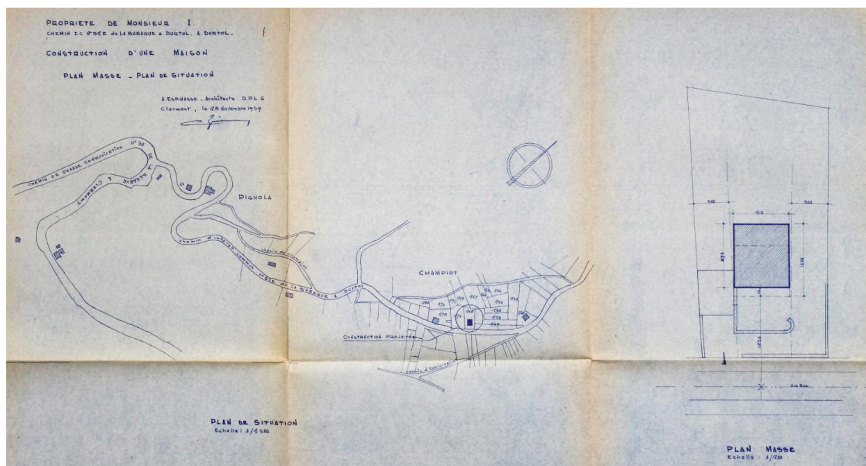
Durtol, la Maison I., plans de masse et de situation, 1959, Antoine Espinasse architecte (Archives municipales de Durtol).
