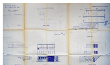
Durtol, la Maison I., coupe et élévations, 1959, Antoine Espinasse architecte (Archives municipales de Durtol). Repro. Christophe Laurent, Autr. Antoine Espinasse IVR84_20216302451NUCA
