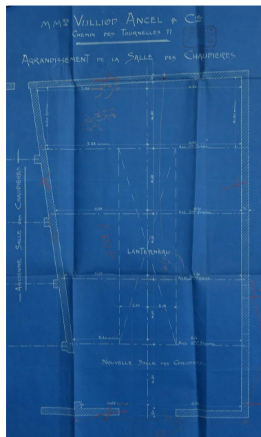
Plan masse, rez-de-chaussée (AC Lyon) Phot. Nadine Halitim-Dubois IVR84_20226901187NUCA
