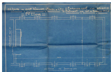
Exhaussement d'un bâtiment, 2e étage, 1912 (AC Lyon : 314W/461-468) Phot. Nadine Halitim-Dubois
