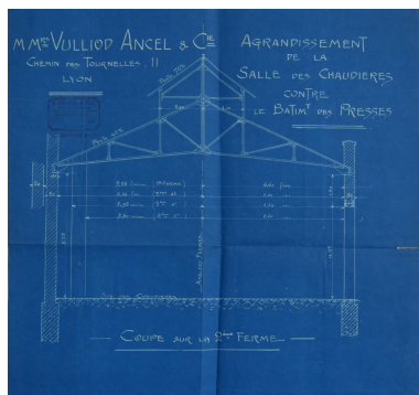
Coupes, élévations (AC Lyon) Phot. Nadine Halitim-Dubois IVR84_20226901186NUCA
