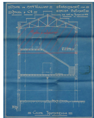
Coupe transversale, exhaussement d'un bâtiment (AC Lyon : 1912, 314W/461 - 468) Phot. Nadine Halitim-Dubois IVR84_20246900079NUCA
