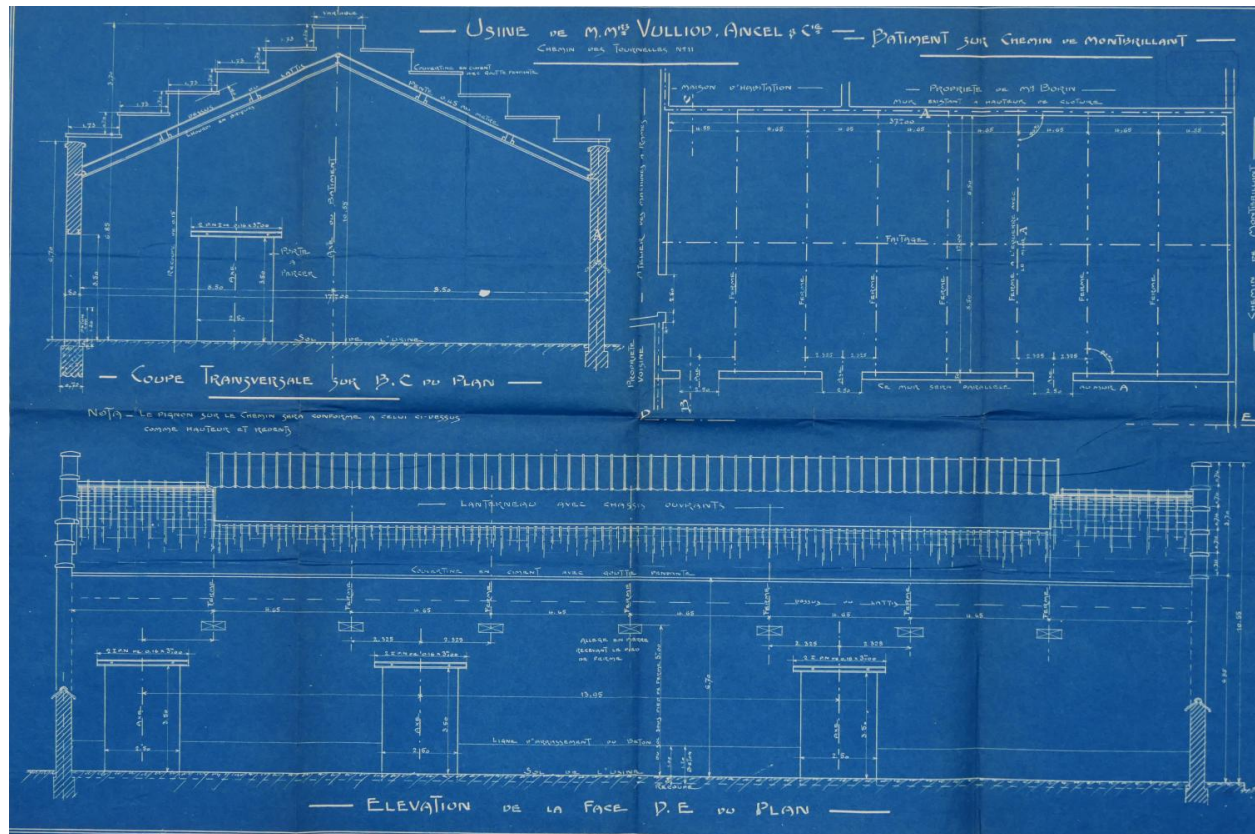
Coupe transversale d'un bâtiment d'usine Vulliot Ancel 1910 (ACL : 314W381-504)
