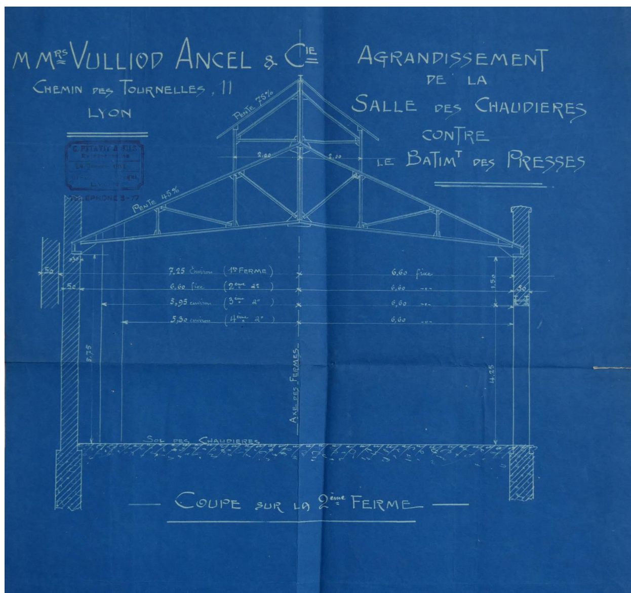
Coupes, élévations (AC Lyon)
