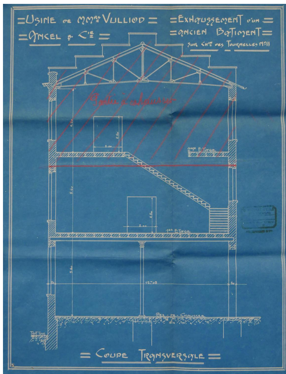
Coupe transversale, exhaussement d'un bâtiment (AC Lyon : 1912, 314W/461 - 468)
