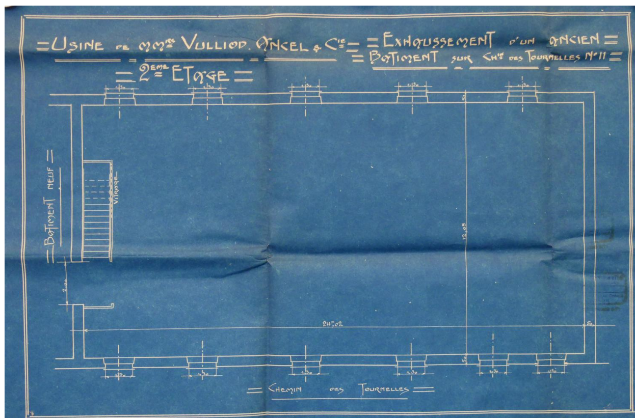
Exhaussement d'un bâtiment, 2e étage, 1912 (AC Lyon : 314W/461-468)
