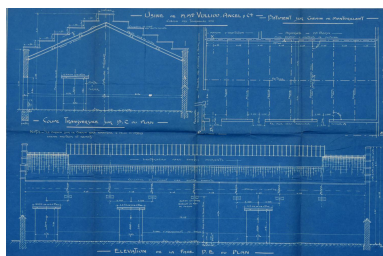
Coupe transversale d'un bâtiment d'usine Vulliot Ancel 1910 (ACL : 314W381-504) Phot. Nadine Halitim-Dubois IVR84_20246900092NUCA
