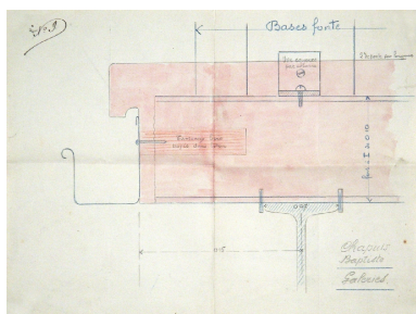
Détail d'exécution des galeries Repro. François Fouger IVR82_20047300243NUCB
