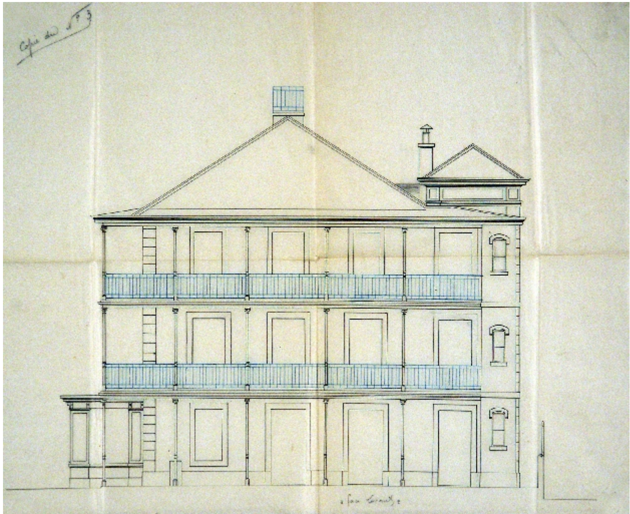
Elévation orientale de la villa
