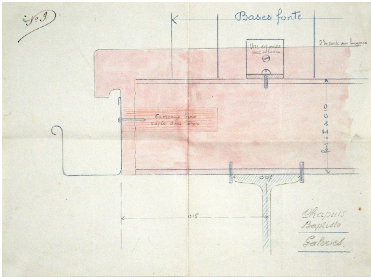
Détail d'exécution des galeries
