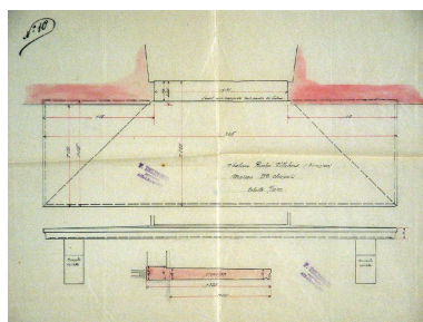
Détail d'exécution des balcons Repro. François Fouger IVR82_20047300244NUCB
