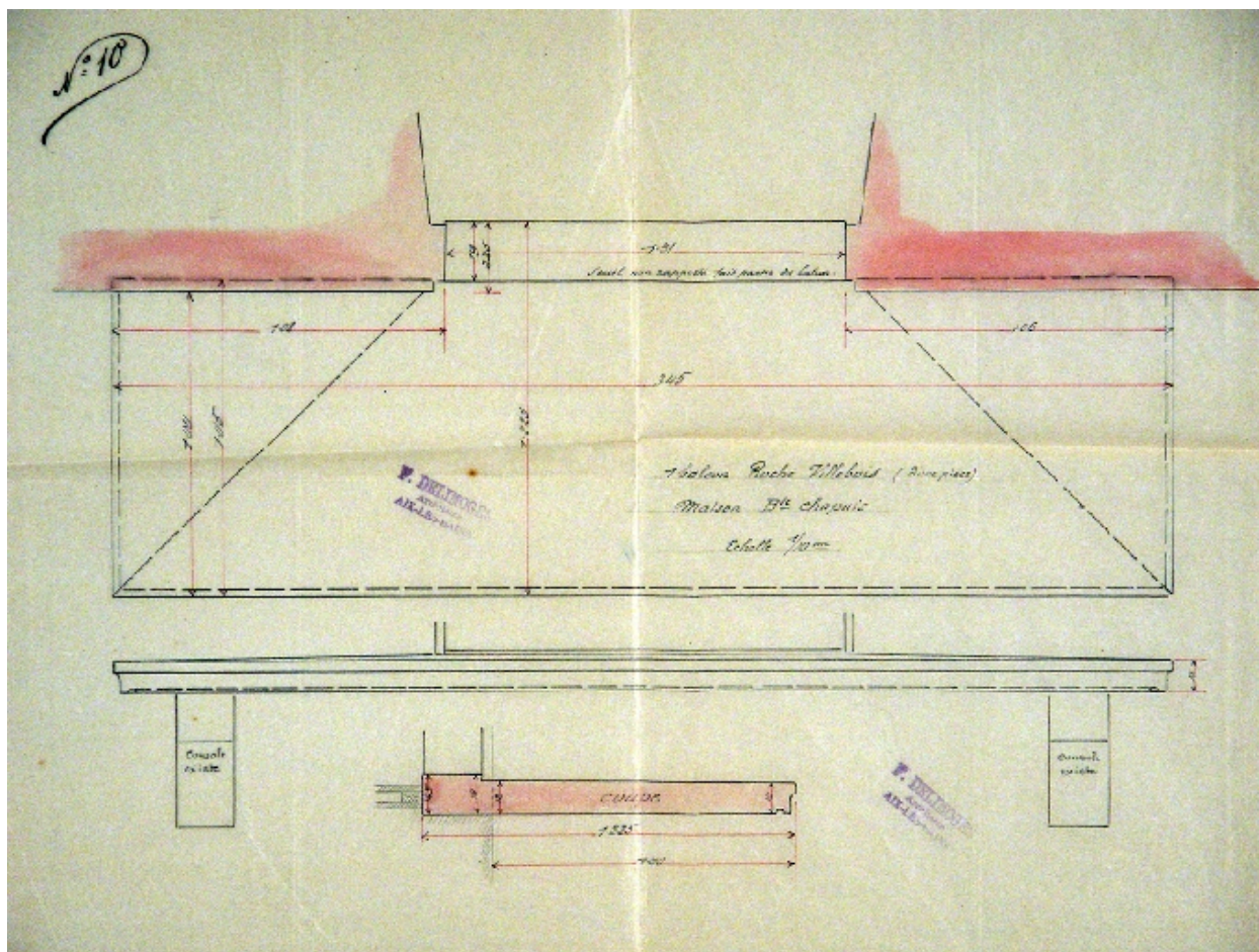
Détail d'exécution des balcons
