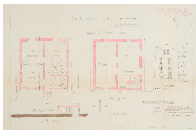
Plans et élévation Repro. François Fouger IVR82_20097301059NUCB
