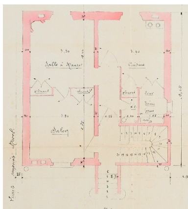
Plan du rez-de-chaussée Repro. François Fouger IVR82_20097301061NUCB
