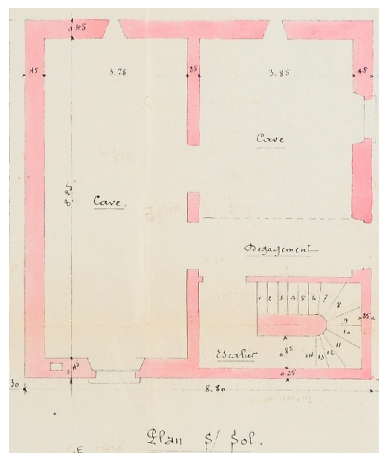
Plan du sous-sol Repro. François Fouger IVR82_20097301062NUCB
