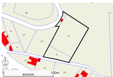
Plan de situation, sur fond de plan cadastral, section AH, échelle originale 1:1250. Source : Direction générale des Finances Publiques - Cadastre ; mise à jour : 1986 Dess. Thierry Monnet
