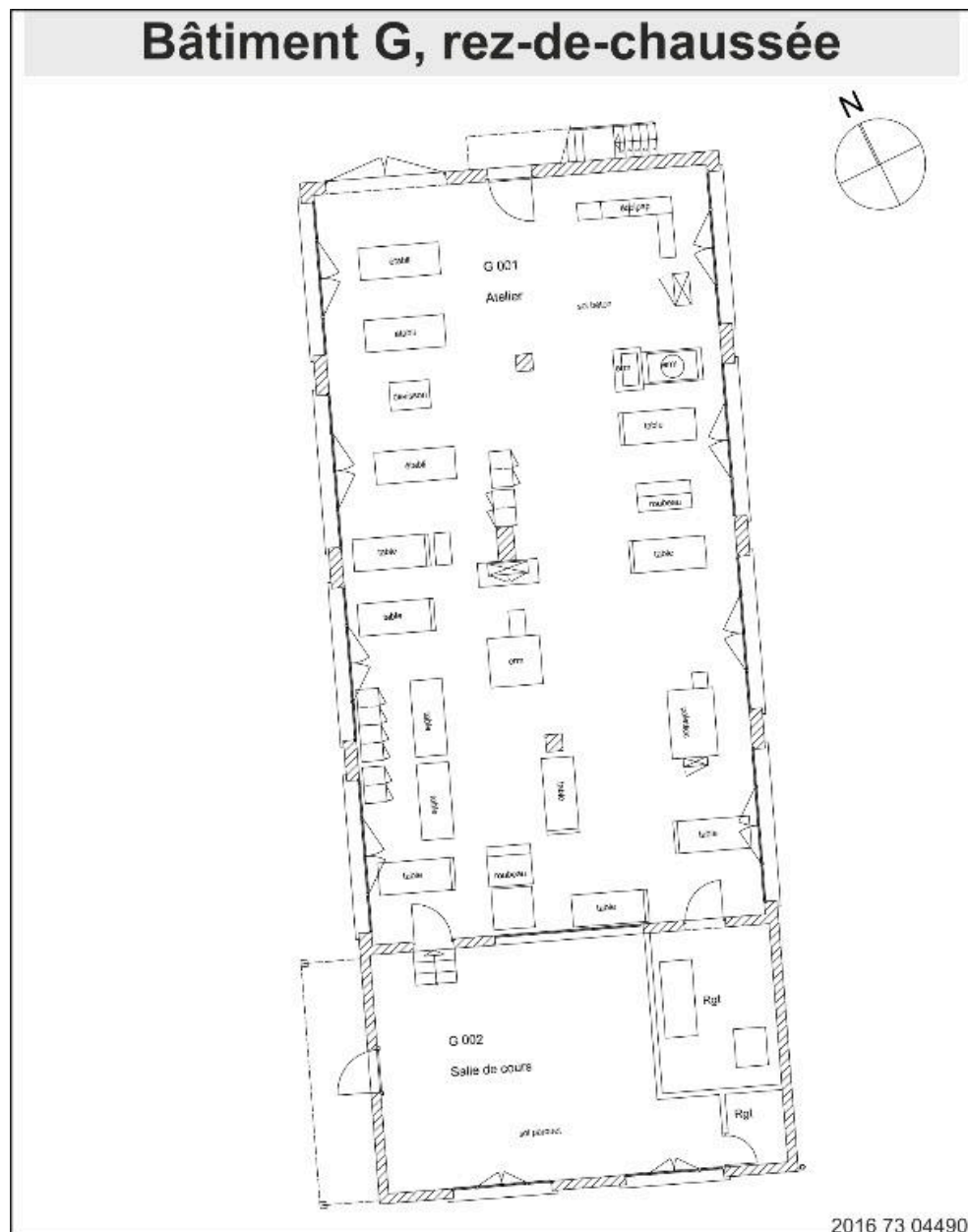
Bâtiment G, rez-de-chaussée
