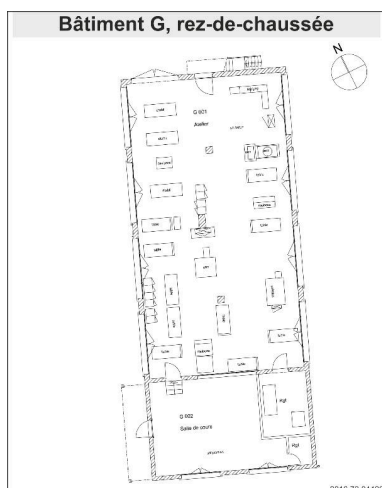
Bâtiment G, rez-de-chaussée Autr. AGATE, géomètres-experts, Dess. André Céréza IVR84_20167304490NUDA
