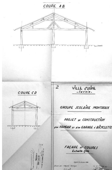
Groupe scolaire. Projet de construction d'un hangar et d'un garage à bicyclettes, Coupes (AD Savoie, 1 Z 481) Repro. Catherine Guégan IVR84_20167304333NUCA
