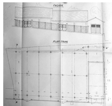
Groupe scolaire. Projet de construction d'un hangar et d'un garage à bicyclettes, Coupes et façades (AD Savoie, 1 Z 481) Repro. Catherine Guégan IVR84_20167304334NUCA
