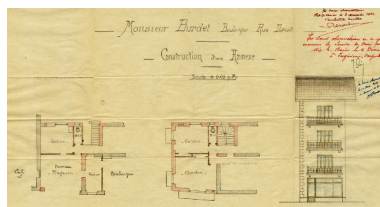
Construction d'une annexe, plans et élévation Repro. François Fouger IVR82_20037300069NUCB
