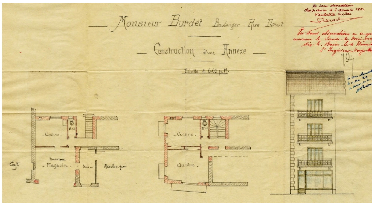
Construction d'une annexe, plans et élévation
