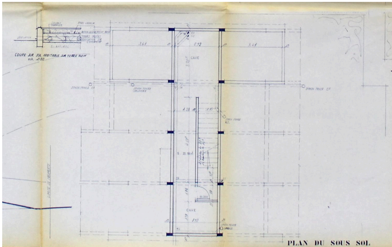
Romagnat, la maison B., plan du sous-sol, Lucien Ambrosetti et J.-P. Gauer architectes, juin 1969 (archives municipales de Romagnat).
