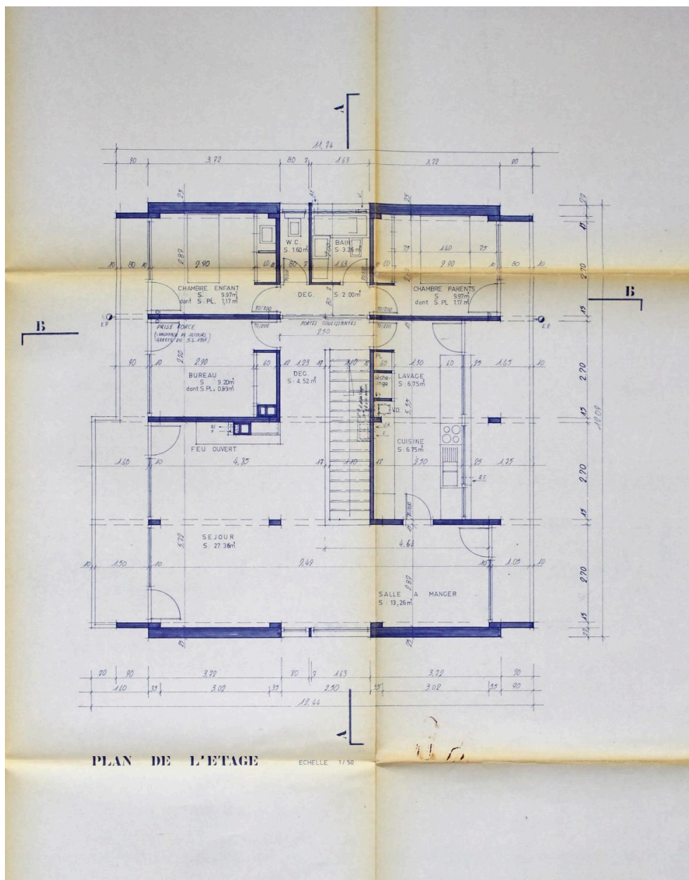
Romagnat, la maison B., plan de l'étage, Lucien Ambrosetti et J.-P. Gauier architectes, juin 1969 (archives municipales de Romagnat).
