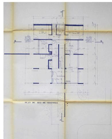
Romagnat, la maison B., plan du rez-de-chaussée, Lucien Ambrosetti et
