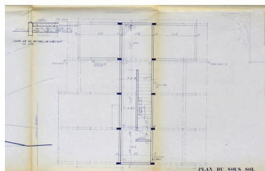
Romagnat, la maison B., plan du sous-sol, Lucien Ambrosetti et J.-P. Guier architectes, juin 1969 (archives municipales de Romagnat). Phot. Lucien AMBROSETTI, Phot. J.-P. GAUER, Phot. Christophe Laurent IVR84_20246301931NUCA
