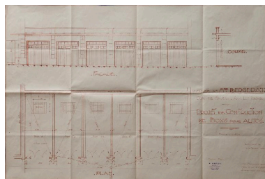
Plan et élévation des garages, 1935 Repro. Denys Harreau IVR82_20147301118NUCB
