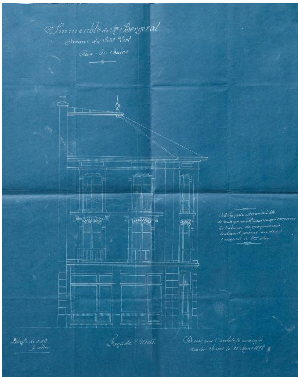
Façade sud de l'immeuble, 1898
