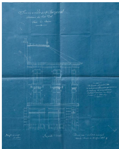
Façade sud de l'immeuble, 1898 Repro. Denys Harreau IVR82_20147301119NUCB
