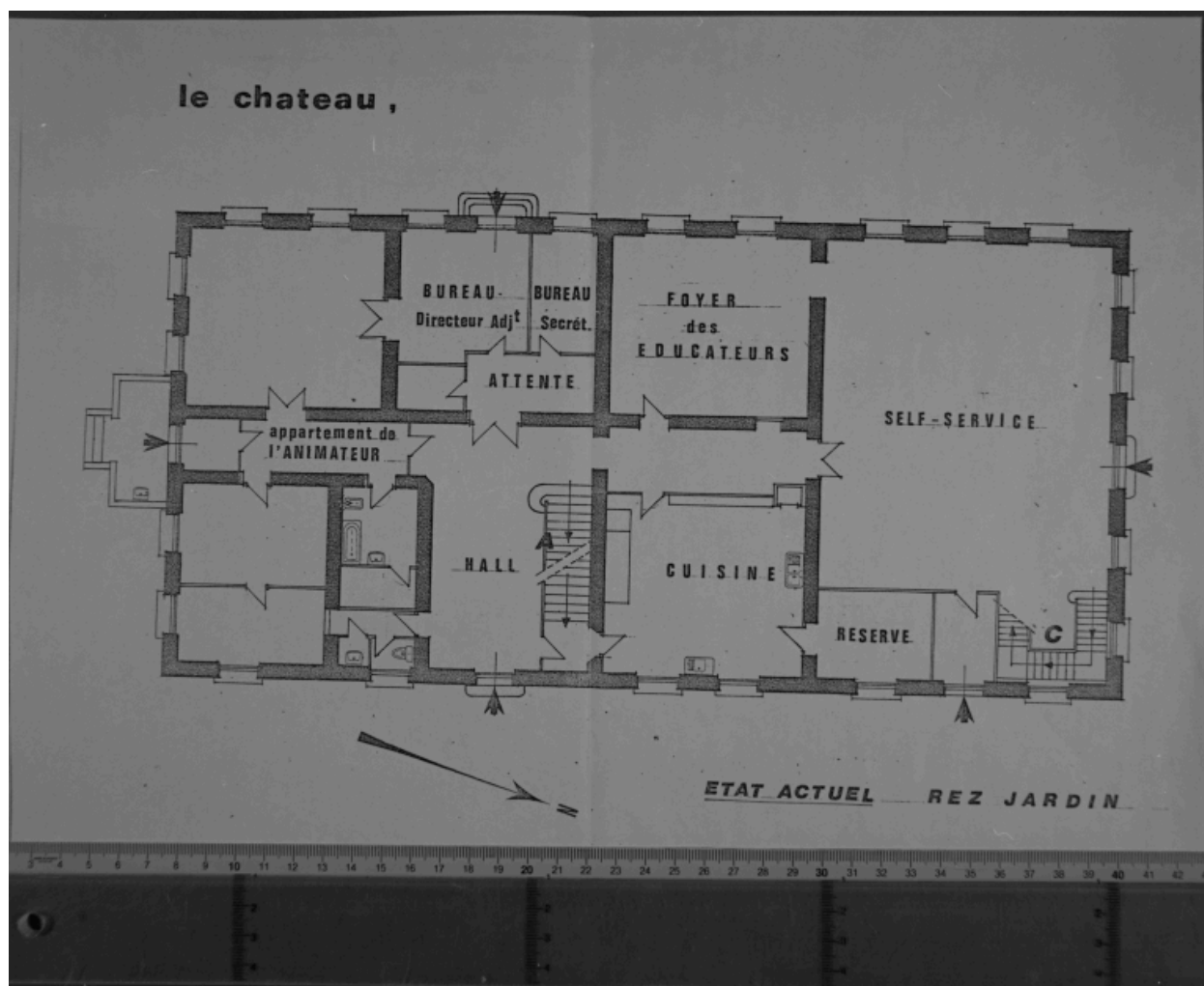
Le château. Etat actuel. Rez-jardin. Plan du rez-de-chaussée, par Abel Cholat, architecte, 1978, [éch. 1/100]
