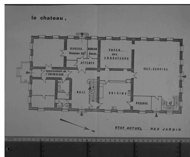
Le château. Etat actuel. Rez-jardin. Plan du rez-de-chaussée, par Abel Cholat, architecte, 1978, [éch. 1/100] Repro. Jean-Marie Refflé, Autr. Abel (architecte) Cholat IVR82_19960100043X
