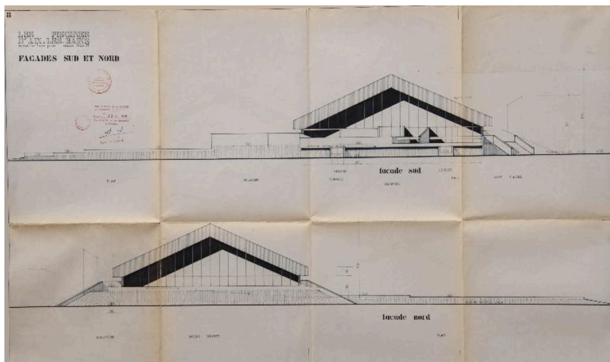
Façades nord et sud, 1971
