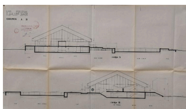
Coupes, 1971 Repro. Denys Harreau IVR82_20157300760NUCB
