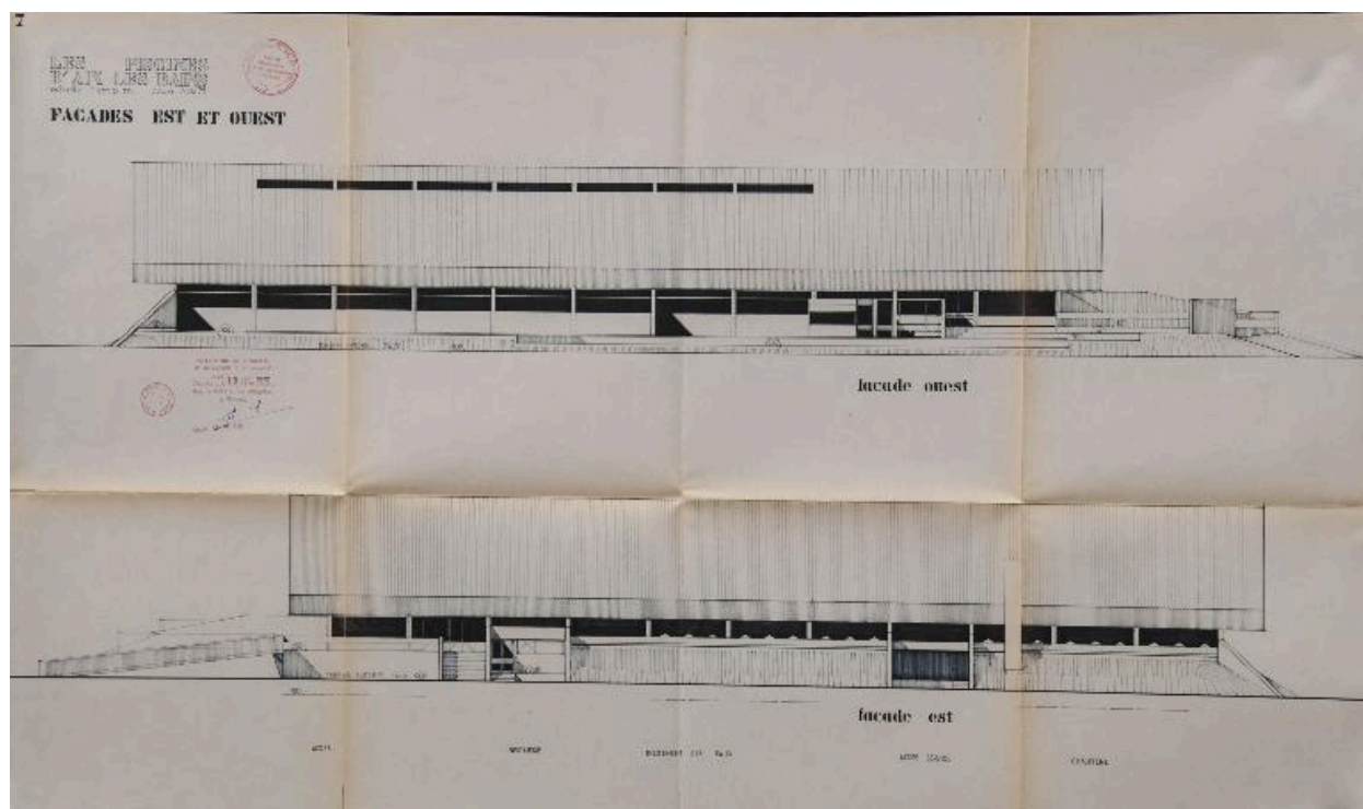
Façades est et ouest, 1971
