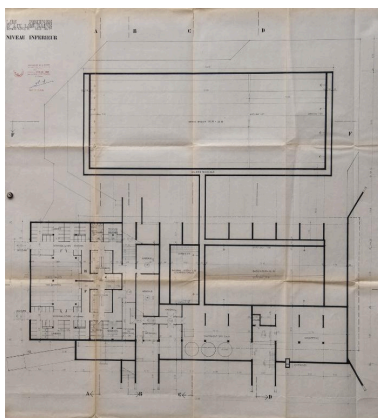
Plan du niveau inférieur, 1971 Repro. Denys Harreau IVR82_20157300758NUCB
