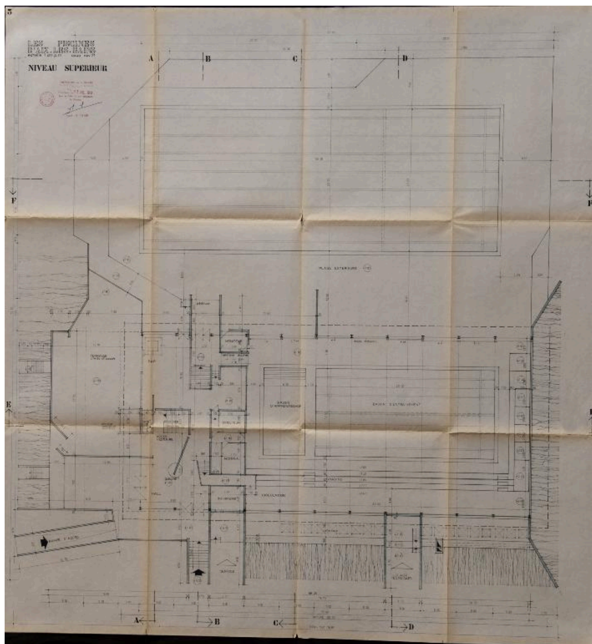
Plan du niveau supérieur, 1971
