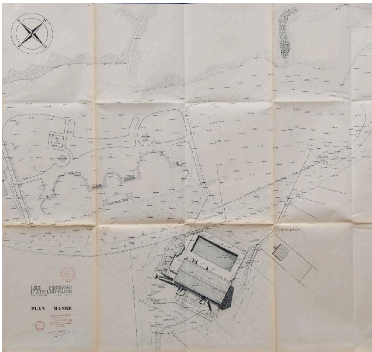
Plan masse, 1971
