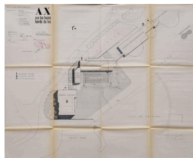
Projet non réalisé, 1970 : plan masse Repro. Denys Harreau IVR82_20157300754NUCB
