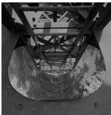
Vue plongeante à travers les arceaux de protection de l'échelle de l'éolienne. Phot. Eric Dessert IVR82_20014201615X
