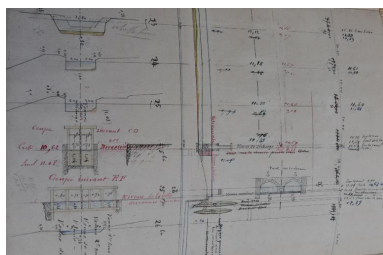
Schéma des roues, 1874 (FR.AD073, 49SPC2). Autr. Clara Bérelle IVR82_20157301742NUCA
