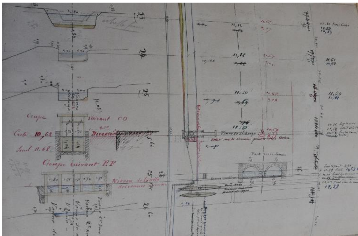
Shéma des roues, 1874 (FR.AD073, 49SPC2).
