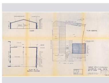
Plans et coupe Repro. François Fouger IVR82_20087300319NUCB
