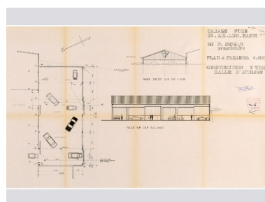
Plan et élévations de l'atelier Repro. François Fouger IVR82_20087300318NUCB
