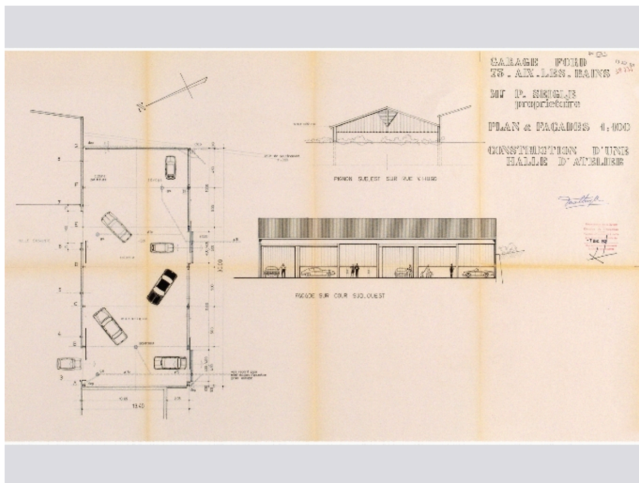
Plan et élévations de l'atelier
