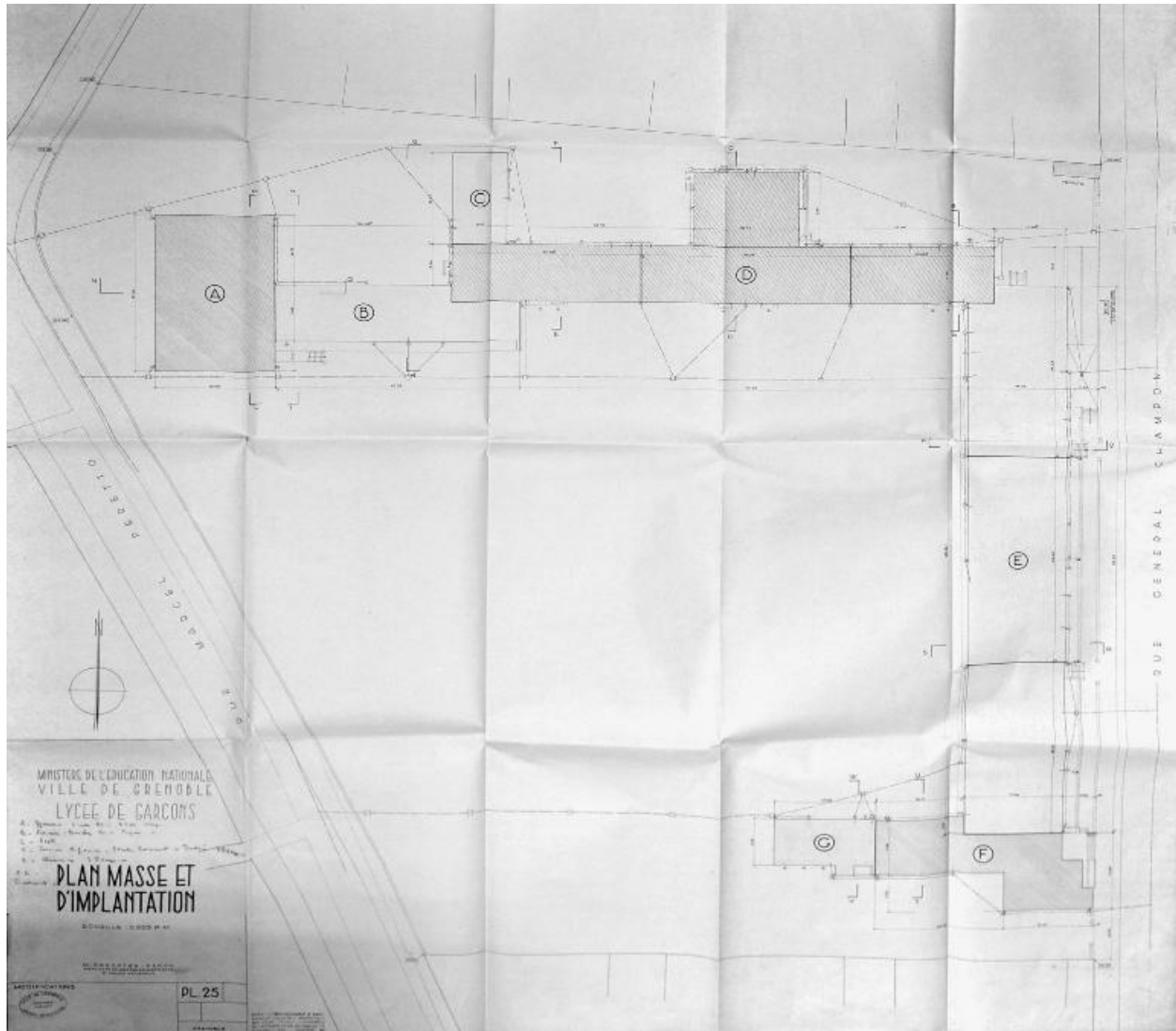
Plan masse et d'implantation, par M. Descote-Genon, 10.4.1958 (AC Grenoble, 4 M 89)
