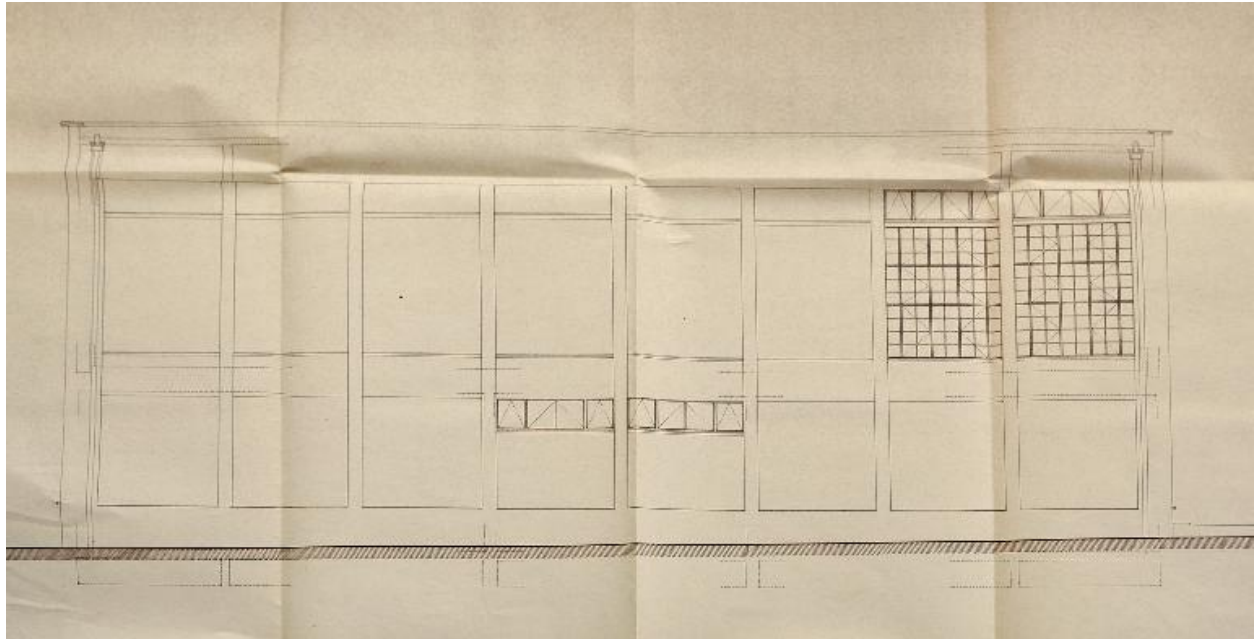
Bâtiment A. Façade ouest, par M. Descote-Genon, 10.4.1958 (AC Grenoble, 4 M 89)
