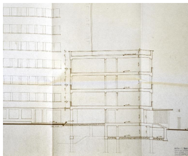
Bâtiments A-B-D. Façade sud, coupe PQ au bâtiment E, par M. Descote-Genon, 10.4.1958 : détail partie droite (AC Grenoble, 4 M 89) Repro. Catherine Guégan, Autr. Marcel-Benoît-Auguste Descotes-Genon IVR84_20163800217NUCA
