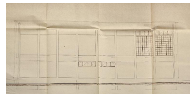
Bâtiment A. Façade ouest, par M. Descote-Genon, 10.4.1958 (AC Grenoble, 4 M 89) Repro. Catherine Guégan, Autr. Marcel-Benoît-Auguste Descotes-Genon IVR84_20163800227NUCA
