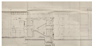
Bâtiments A-B. Façade est, coupe IK, par M. Descote-Genon, 10.4.1958 (AC Grenoble, 4 M 89) Repro. Catherine Guégan, Autr. Marcel-Benoît-Auguste Descotes-Genon IVR84_20163800228NUCA
