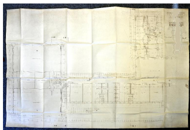
Bâtiments A-B-C, plans du rez-de-chaussée, par M. Descote-Genon, 10.4.1958 (AC Grenoble, 4 M 89) Repro. Catherine Guégan, Autr. Marcel-Benoît-Auguste Descotes-Genon IVR84_20163800220NUCA
