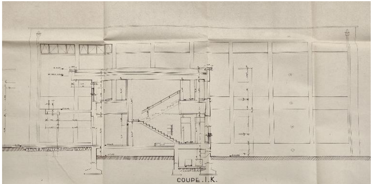
Bâtiments A-B. Façade est, coupe IK, par M. Descote-Genon, 10.4.1958 (AC Grenoble, 4 M 89)
