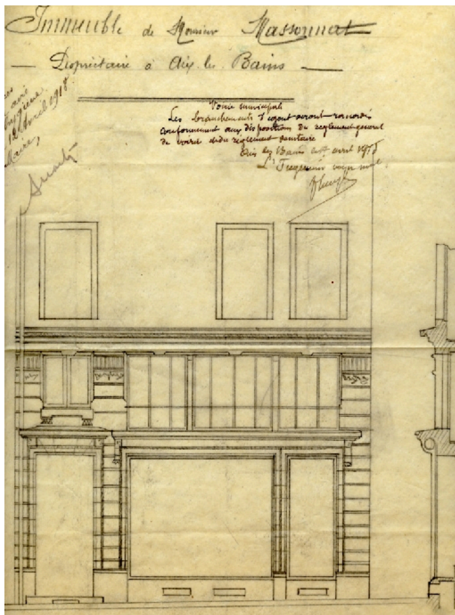
Elévation du rez-de-chaussée
