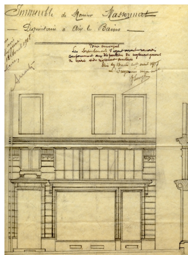
Élévation du rez-de-chaussée Repro. François Fouger IVR82_20057300934NUCB
