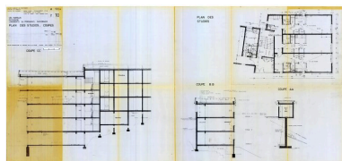
Extension logements personnel saisonnier. Plan et coupe d'un studio / Atelier d'architecture en Montagne, 2 mars 1984 (AC Montricher-Albanne) Phot. Jean-François Lyon-Caen IVR82_20127302410NUC
