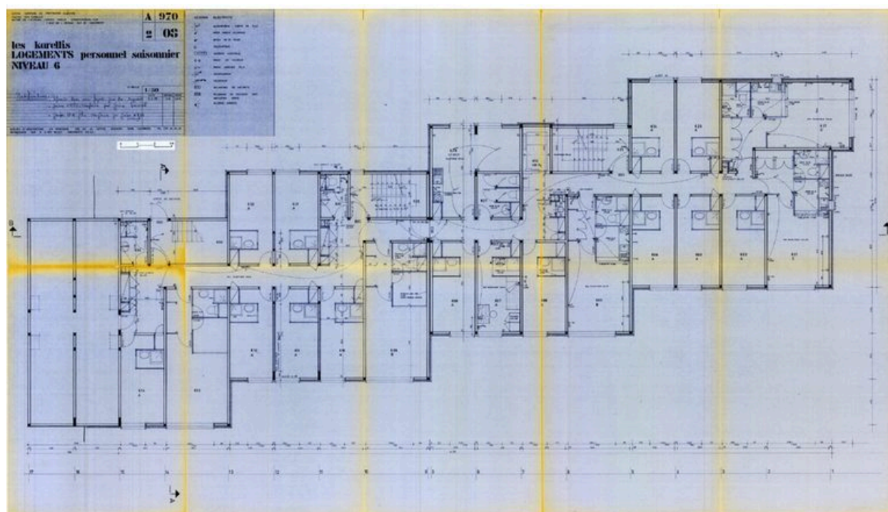
Logements personnel saisonnier. Plan niveau 6 / Atelier d'architecture en Montagne, 9 mars 1978. Modifications 22 juin 1979 (AC Montricher-Albanne)
