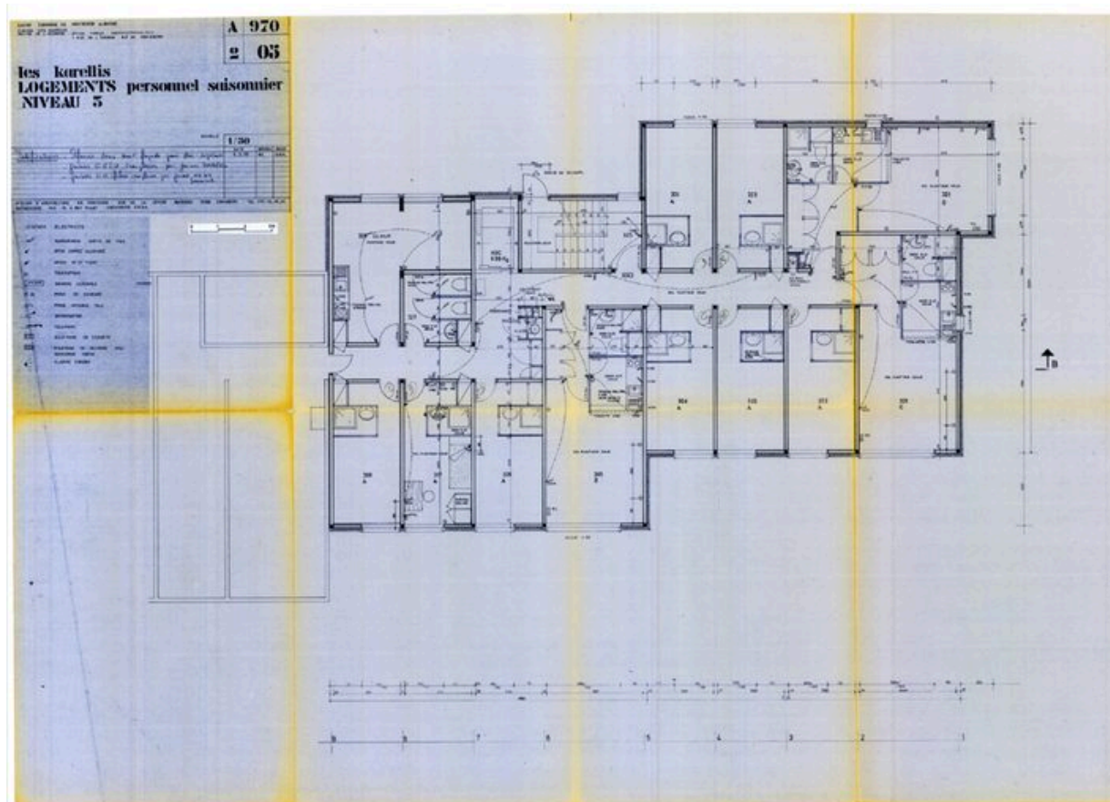
Logements personnel saisonnier. Plan niveau 3 / Atelier d'architecture en Montagne, 9 mars 1978. Modifications 22 juin 1979 (AC Montricher-Albanne)
