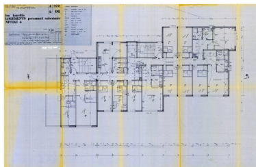
Logements personnel saisonnier. Plan niveau 4 / Atelier d'architecture en Montagne, 9 mars 1978. Modifications 22 juin 1979 (AC Montricher-Albanne) Phot. Jean-François Lyon-Caen IVR82_20127302405NUC
