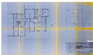
Logements personnel saisonnier. Plan niveau 0 et 1 / Atelier d'architecture en Montagne, 9 mars 1978. Modifications 22 juin 1979 (AC Montricher-Albanne) Phot. Jean-François Lyon-Caen IVR82_20127302402NUC
