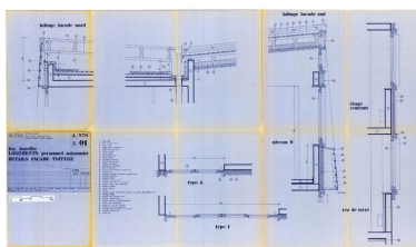
Logements personnel saisonnier. Détails de façade et de toiture / Atelier d'architecture en Montagne, 9 mars 1978. Modifications 22 juin 1979 (AC Montricher-Albanne) Phot. Jean-François Lyon-Caen IVR82_20127302408NUC
