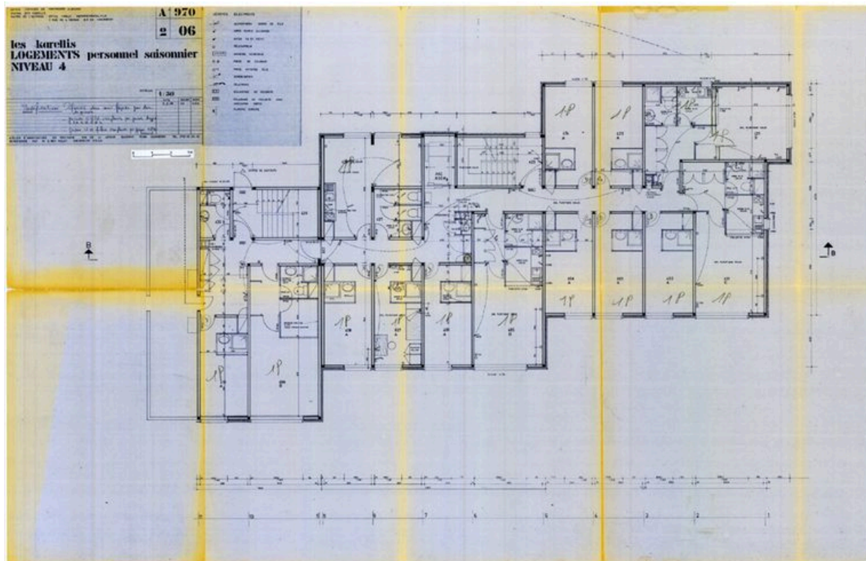
Logements personnel saisonnier. Plan niveau 4 / Atelier d'architecture en Montagne, 9 mars 1978. Modifications 22 juin 1979 (AC Montricher-Albanne)
