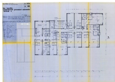
Logements personnel saisonnier. Plan niveau 3 / Atelier d'architecture en Montagne, 9 mars 1978. Modifications 22 juin 1979 (AC Montricher-Albanne) Phot. Jean-François Lyon-Caen IVR82_20127302404NUC
