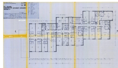
Logements personnel saisonnier. Plan niveau 5 / Atelier d'architecture en Montagne, 9 mars 1978. Modifications 22 juin 1979 Phot. Jean-François Lyon-Caen IVR82_20127302406NUC
