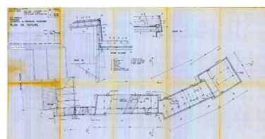
Extension logements personnel saisonnier. Plan de toiture / Atelier d'architecture en Montagne, 2 mars 1984 (AC Montricher-Albanne) Phot. Jean-François Lyon-Caen IVR82_20127302409NUC
