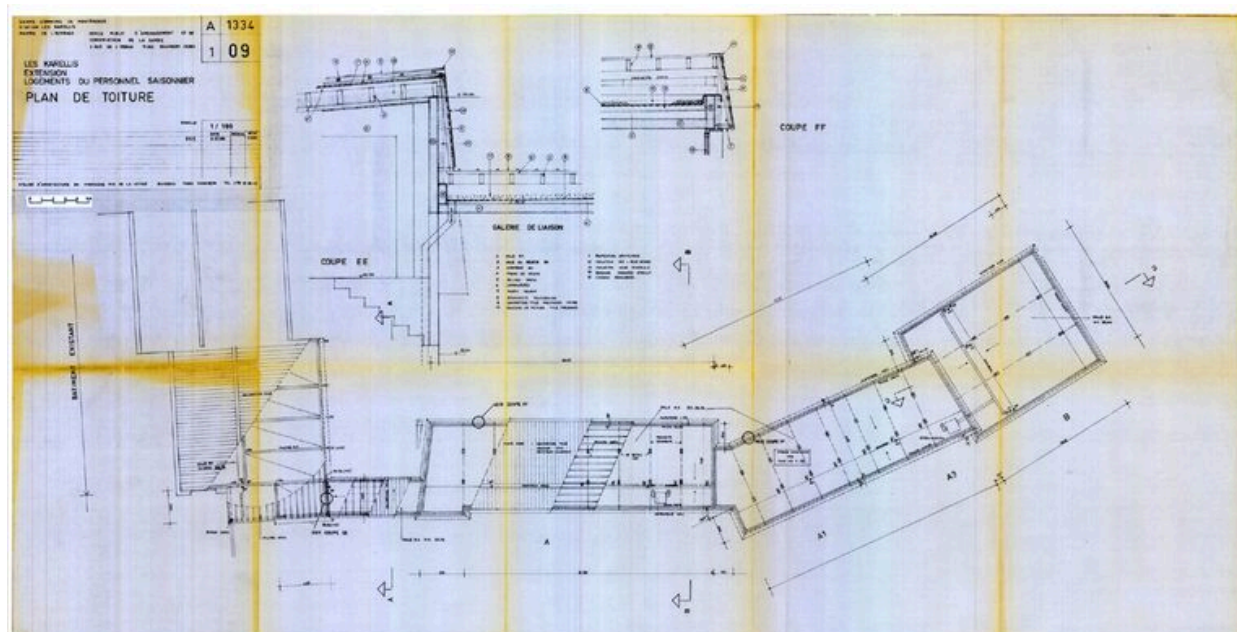
Extension logements personnel saisonnier. Plan de toiture / Atelier d'architecture en Montagne, 2 mars 1984 (AC Montricher-Albanne)
