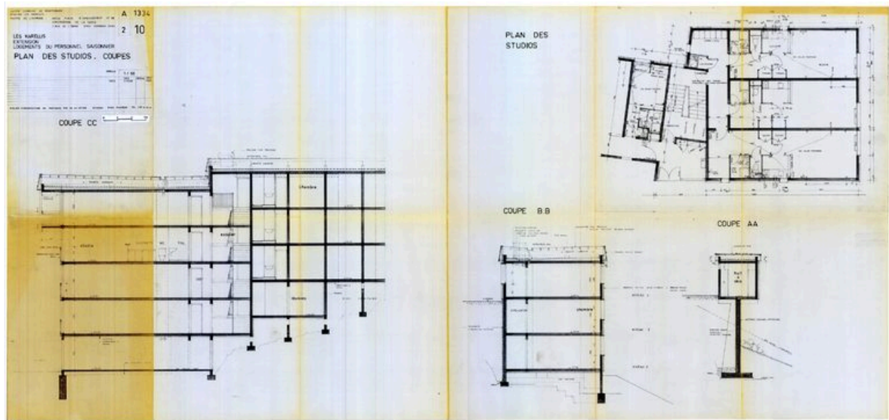
Extension logements personnel saisonnier. Plan et coupe d'un studio / Atelier d'architecture en Montagne, 2 mars 1984 (AC Montricher-Albanne)
