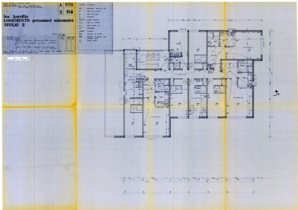
Logements personnel saisonnier. Plan niveau 2 / Atelier d'architecture en Montagne, 9 mars 1978. Modifications 22 juin 1979 (AC Montricher-Albanne)
