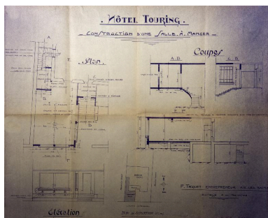
Construction de la salle à manger, 1930 : plans, coupes et élévation Repr. Denys Harreau IVR84_20177300252NUCB
