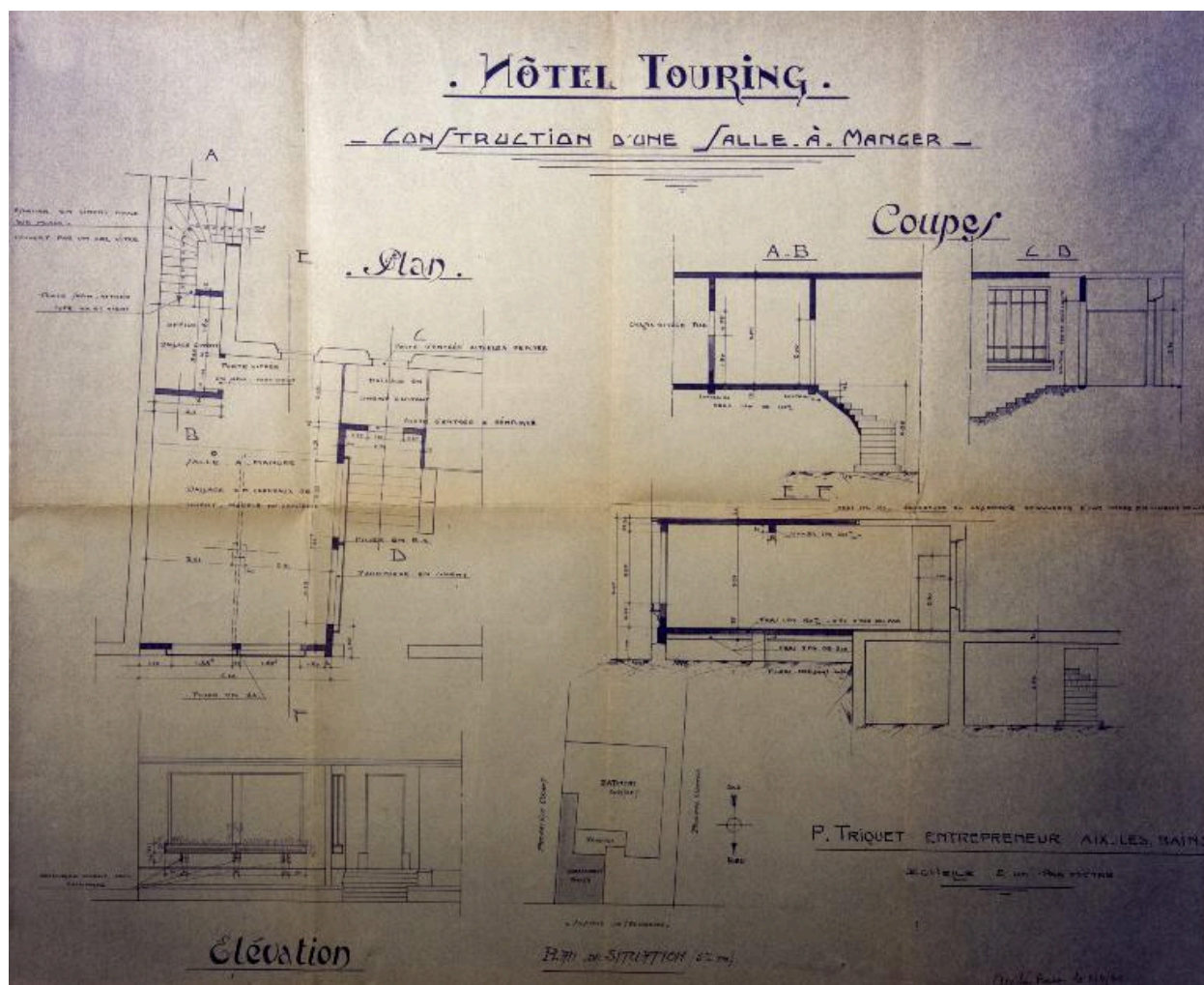
Construction de la salle à manger, 1930 : plans, coupes et élévation
