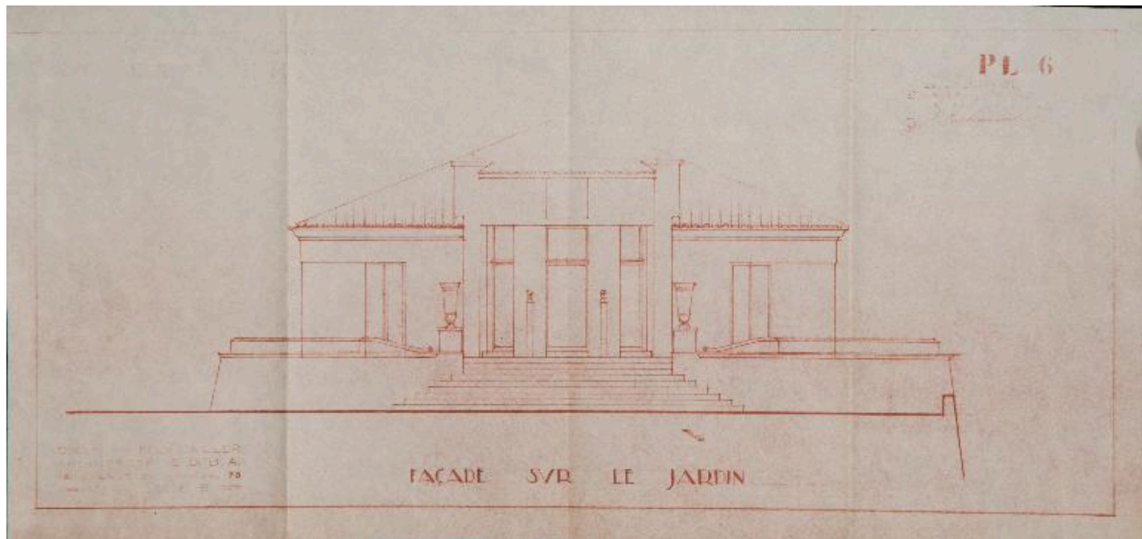
Façade sur jardin, 1934
