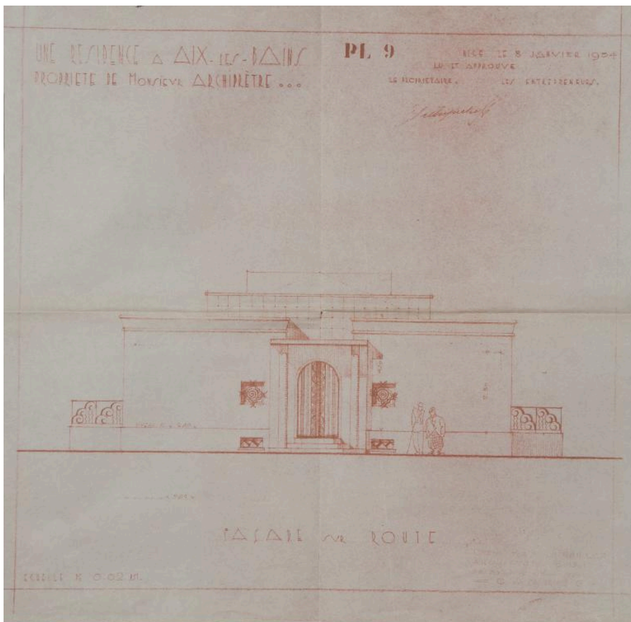
Façade sur route, 1934
