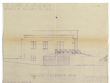
Elévation latérale nord, 1933 Repro. François Fouger IVR82_20087300729NUCB
