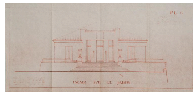
Façade sur jardin, 1934 Repro. Denys Harreau IVR82_20137301005NUCB
