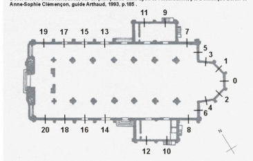
Plan de localisation des verrières du premier niveau Dess. Paul Cherblanc IVR82_20026903670NUD
