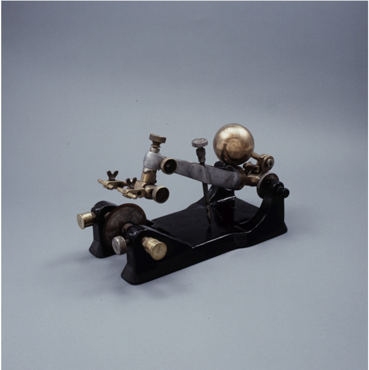
Scie à diamant.
