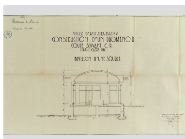
Coupe sur un kiosque Repro. François Fouger IVR82_20067300267NUCB
