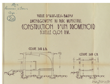
Coupes transversales Repro. François Fouger IVR82_20067300266NUCB
