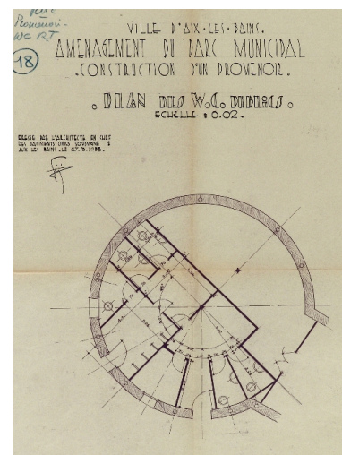
Plan d'un kiosque Repro. François Fouger IVR82_20067300268NUCB
