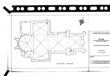
Département de la Loire. Commune de Saint-Laurent-Rochefort. Eglise. Etat des lieux. Plan de l'église." Dessin : J. Mignon, le 20/10/97, échelle originale 1/50e. Phot. Eric Dessert, Autr. J. (architecte) Mignon IVR82_20014200561P
