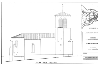
Département de la Loire. Commune de Saint-Laurent-Rochefort. Eglise. Etat des lieux. Façade nord, situation." Dessin : J. Mignon, le 20/10/97, échelle originale 1/50e. Phot. Eric Dessert, Autr. J. (architecte) Mignon IVR82_20014200560P
