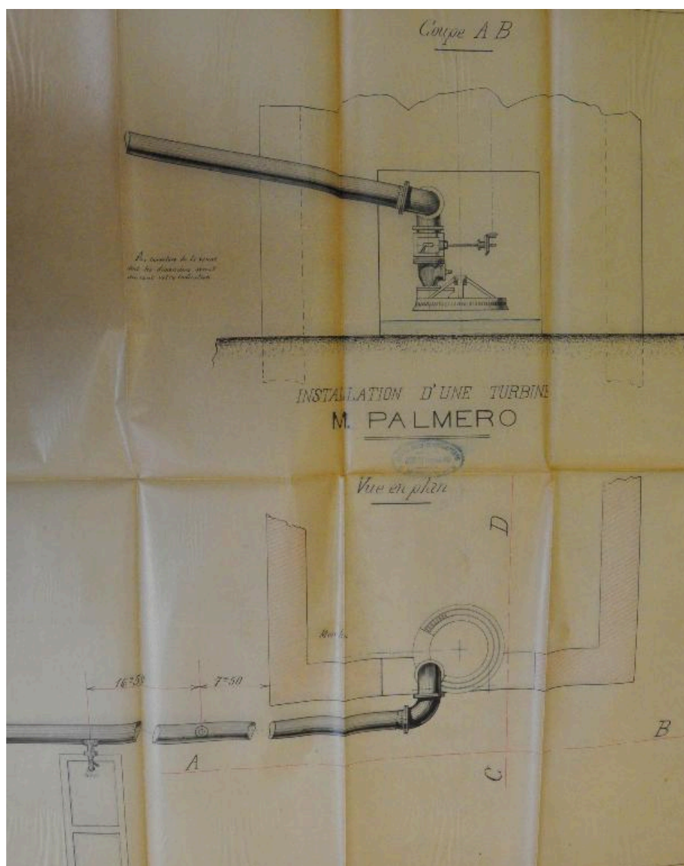
Plan de la conduite et de la turbine de JB.Palmero, 1903 (FR.AD073, 49SPC8).
