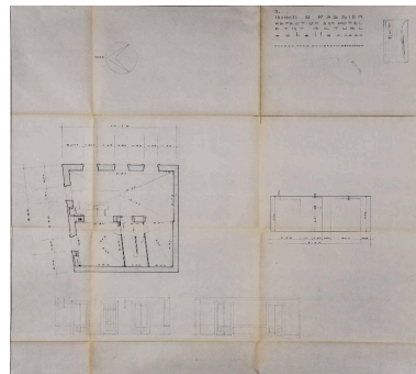
Réfection hôtel, état actuel : plan, élévation, 1960 Repro. Denys Harreau IVR82_20157300274NUCB
