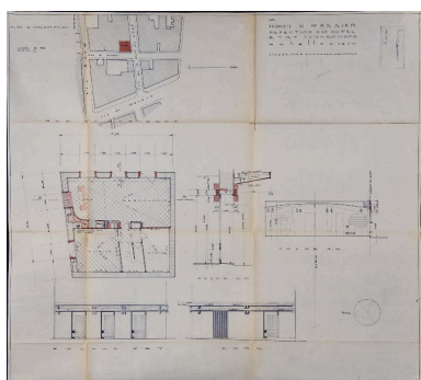
Réfection hôtel, état transformé : plan, élévation et coupe, 1960 Repro. Denys Harreau IVR82_20157300275NUCB
