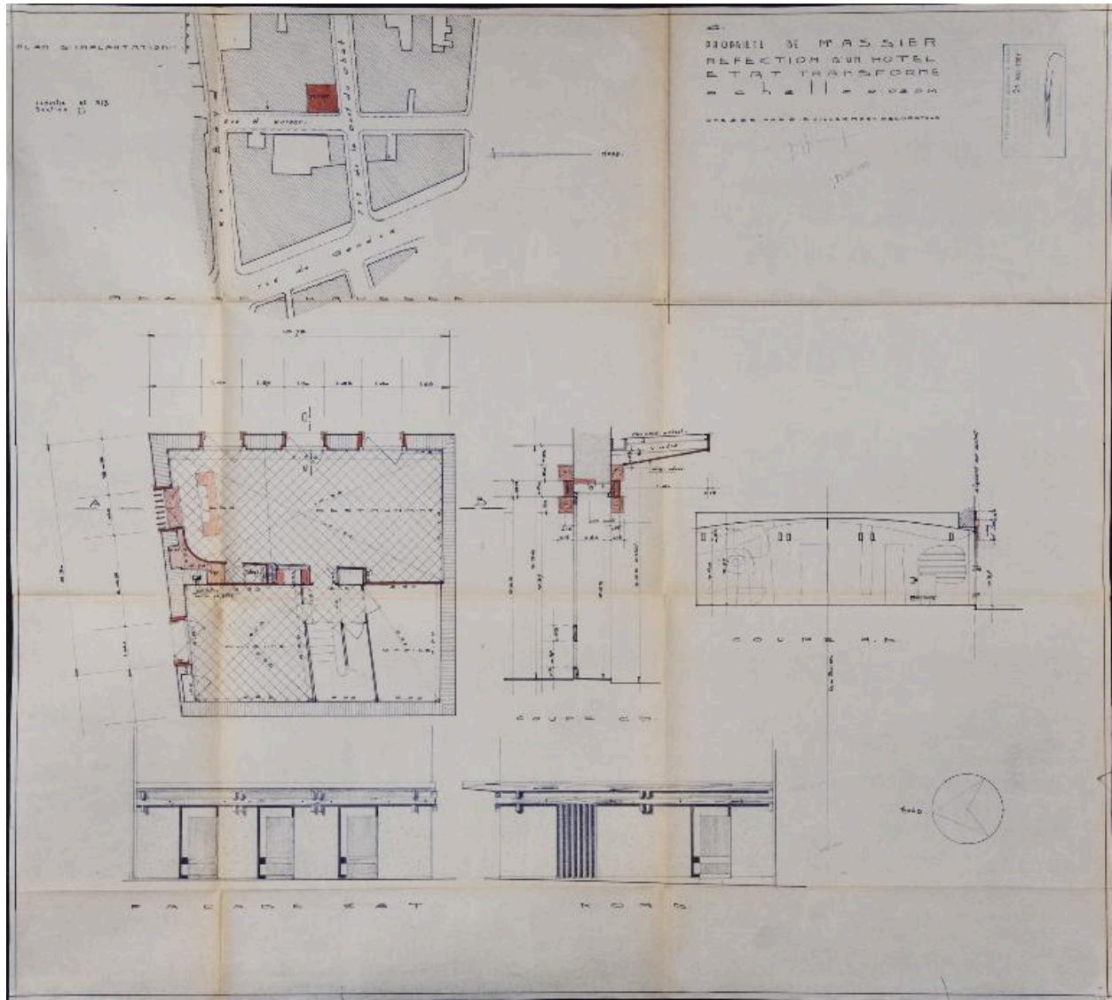
Réfection hôtel, état transformé : plan, élévation et coupe, 1960
