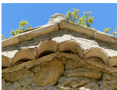
Partie est. Pignon sud, saillie de rive constitué de deux rangs de génoise.
