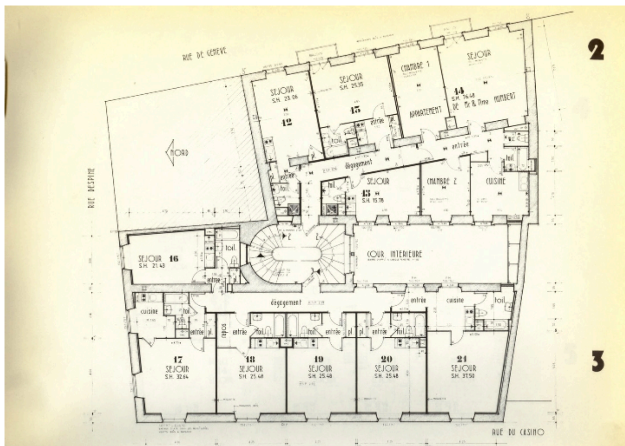
Plan des 2e et 3e étages
