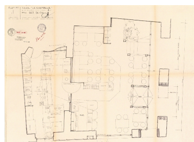
Projet d'aménagement du rez-de-chaussée : plan Repr. François Fouger IVR82_20057302038NUCB
