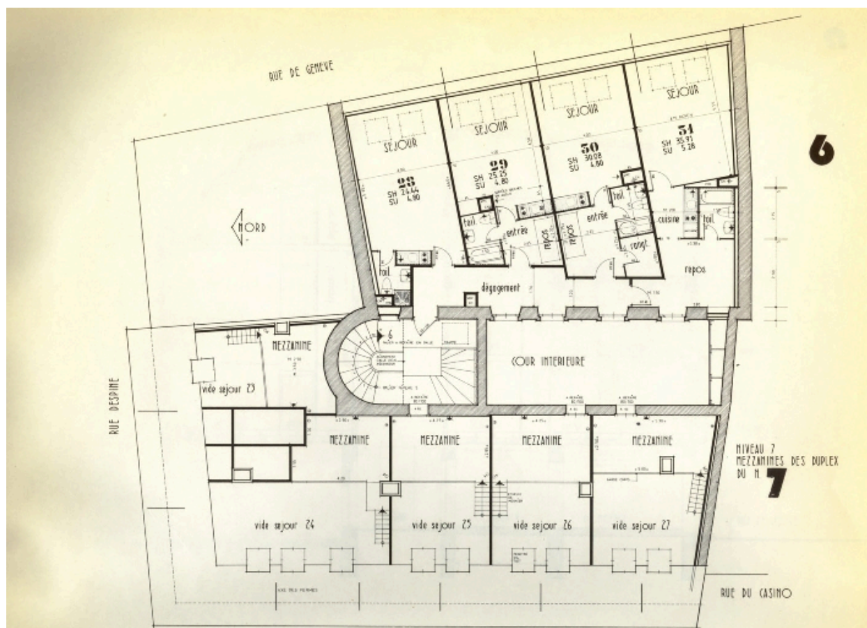
Plan des 6e et 7e étages
