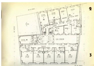
Plan des 2e et 3e étages Repr. François Fouger IVR82_20057300965NUCB
