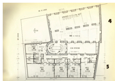
Plan des 4e et 5e étages Repr. François Fouger IVR82_20057300966NUCB
