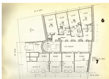
Plan des 6e et 7e étages Repr. François Fouger IVR82_20057300967NUCB
