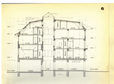
Coupe Repr. François Fouger IVR82_20057300968NUCB
