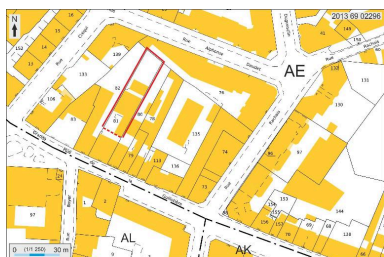
Plan masse et de situation, extrait de http://cadastre.gouv.fr Dess. André Céréza IVR82_20136902296NUDA
