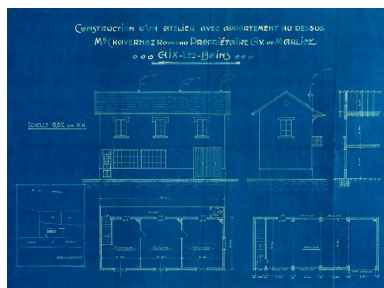
Plans, coupe et élévations Repr. François Fouger IVR82_20087300362NUCB
