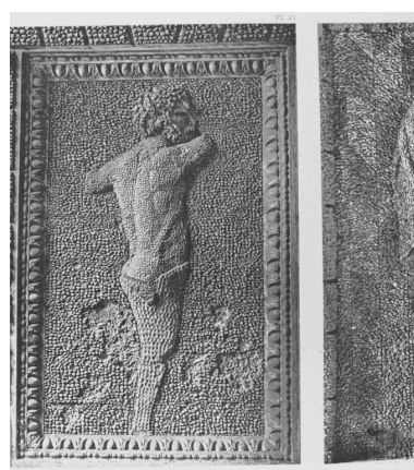
Détail d'un terme ornant le mur est de la grotte et représentant l'été.
