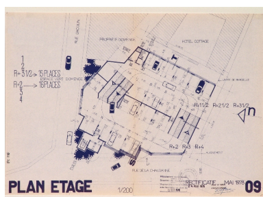
Plan de l'étage Repro. François Fouger IVR82_20057300746NUCB
