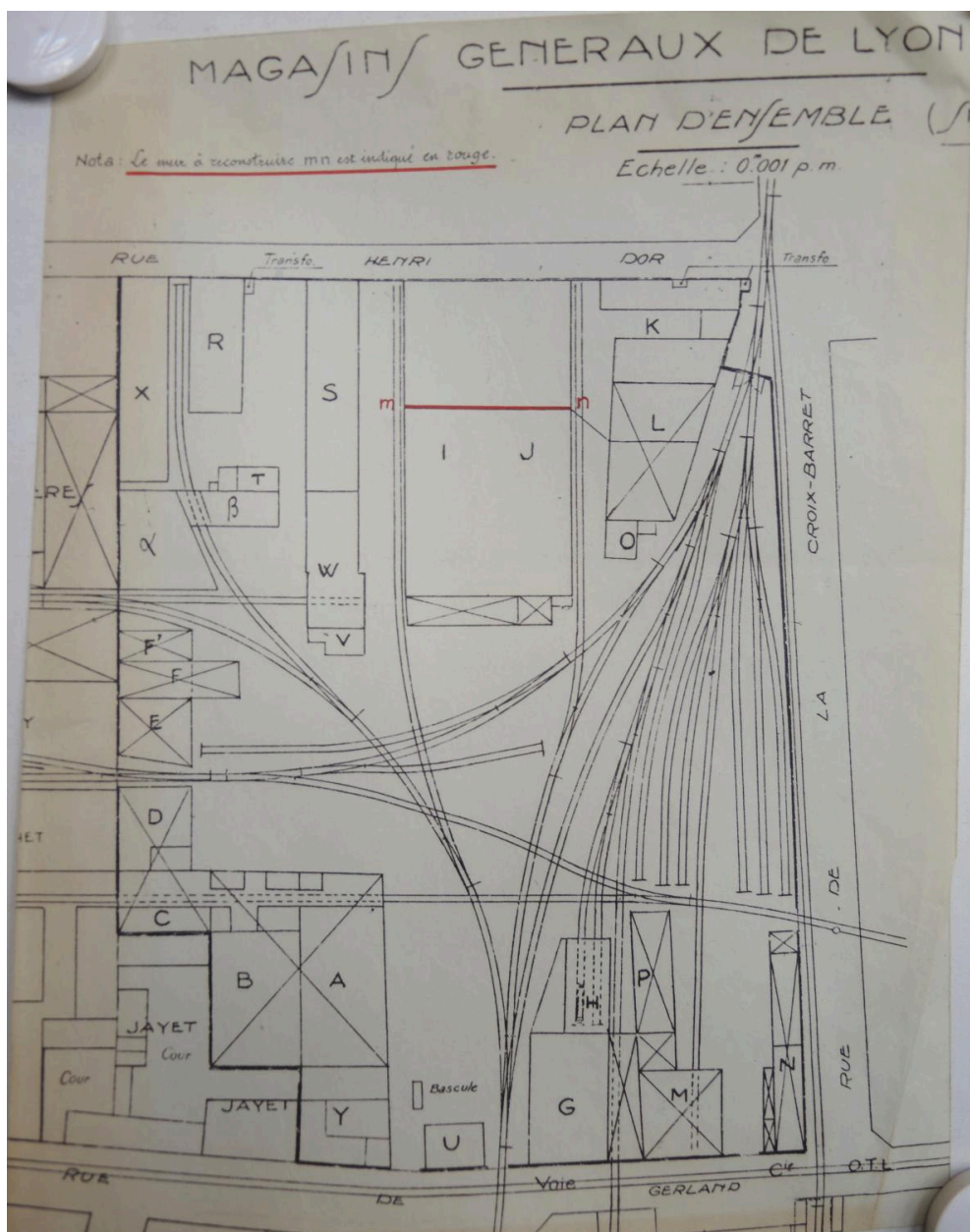
Plan de l'usine avec les raccordements ferroviaires (AC Lyon344w1485, 1944)
