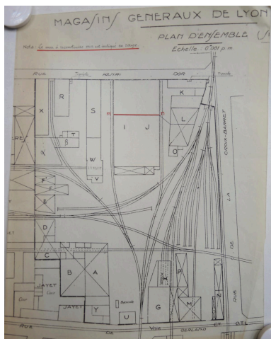
Plan de l'usine avec les raccordements ferroviaires (AC Lyon344w1485, 1944) Phot. Nadine Halitim-Dubois IVR84_20216900118NUCA
