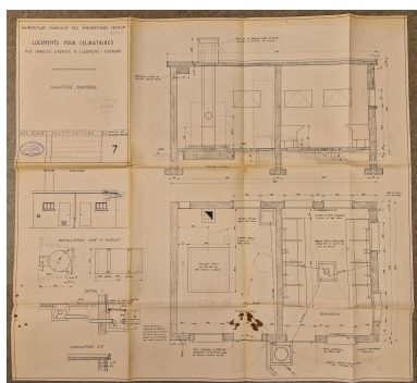
Plan, coupe et détails de la chaufferie-buanderie. Repro. Brigitte Ceroni, Autr. auteur inconnu IVR84_20256301419NUCA
