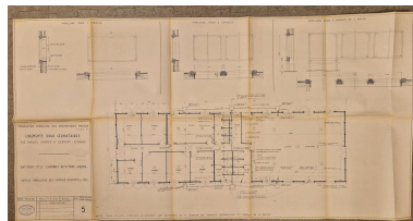
Plan et détails du bâtiment n°2. Repro. Brigitte Ceroni, Autr. auteur inconnu IVR84_20256301417NUCA
