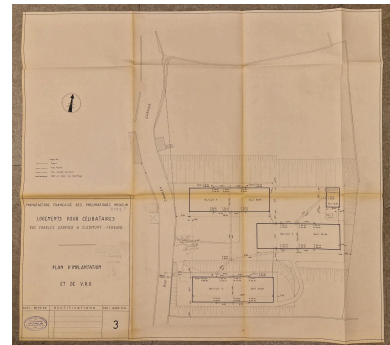
Plan d'implantation et de VRD des différents bâtiments de la cité. Repro. Brigitte Ceroni, Autr. auteur inconnu IVR84_20256301414NUCA
