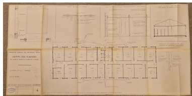
Plan, coupe et détails des bâtiments 1 et 3. Repro. Brigitte Ceroni, Autr. auteur inconnu IVR84_20256301415NUCA
