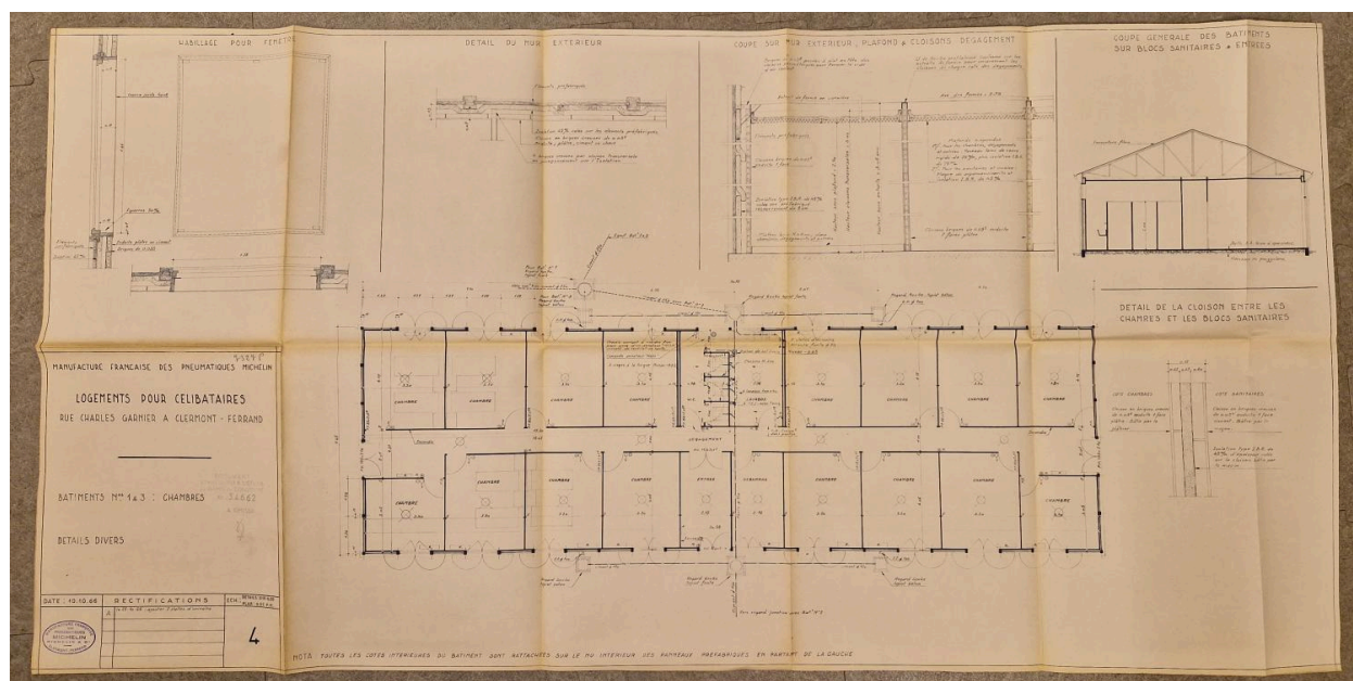
Plan, coupe et détails des bâtiments 1 et 3.
