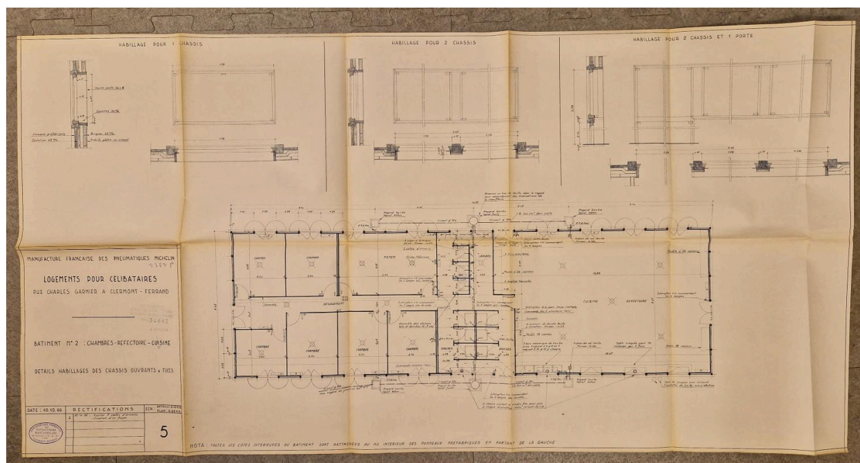
Plan et détails du bâtiment n°2.
