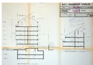
Coupes, 1987 (AC Lyon, 1629 W 034) Repro. Maryannick Chalabi, Autr. Jean-Louis Morlet IVR84_20176901191NUCA
