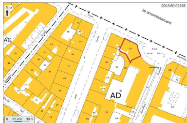
Plan masse et de situation, extrait de http://cadastre.gouv.fr Dess. André Céréza IVR82_20136902176NUDA
